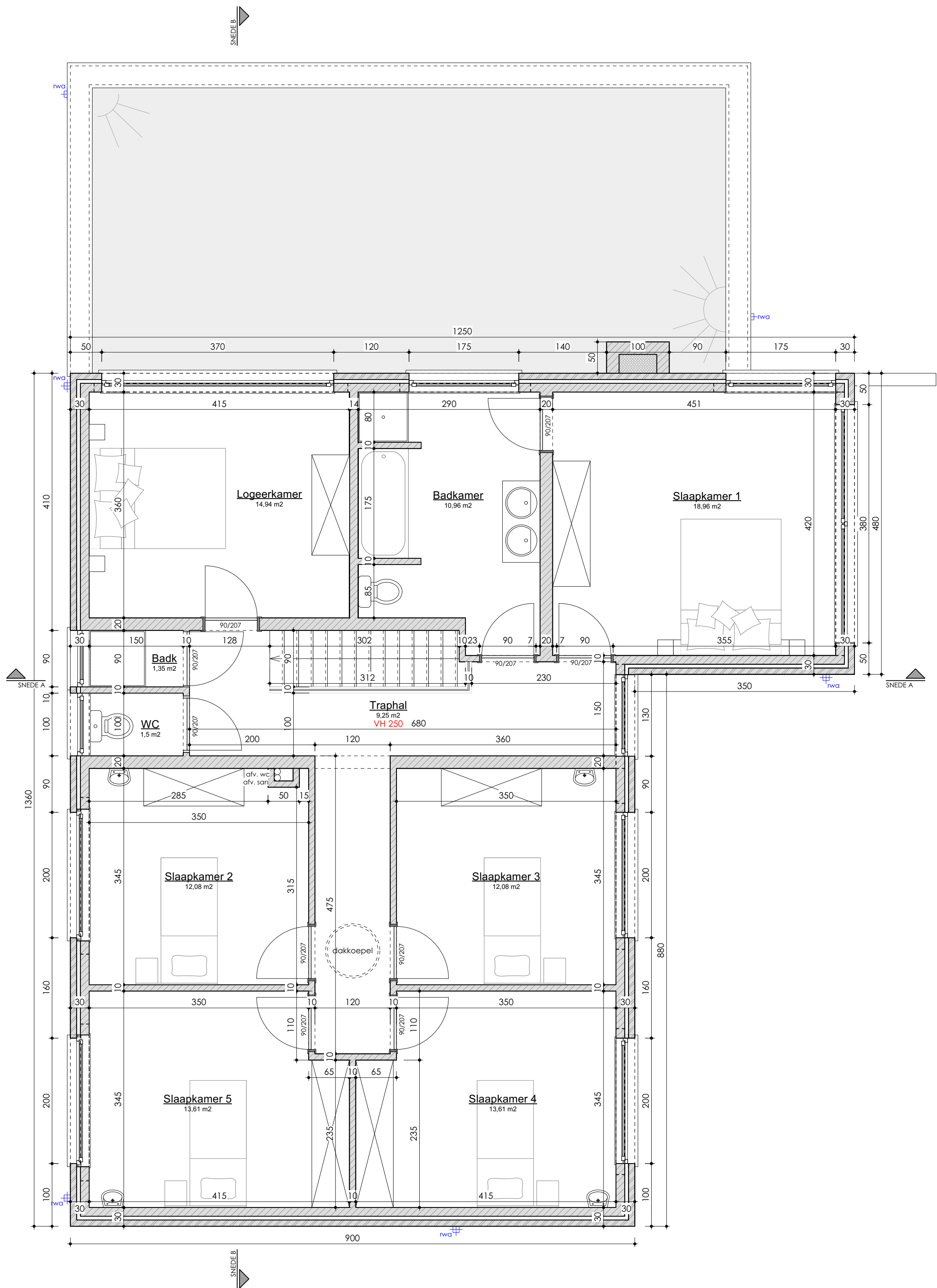
Verdiepingsplan -Bestaande toestand Schaal: 1:50
