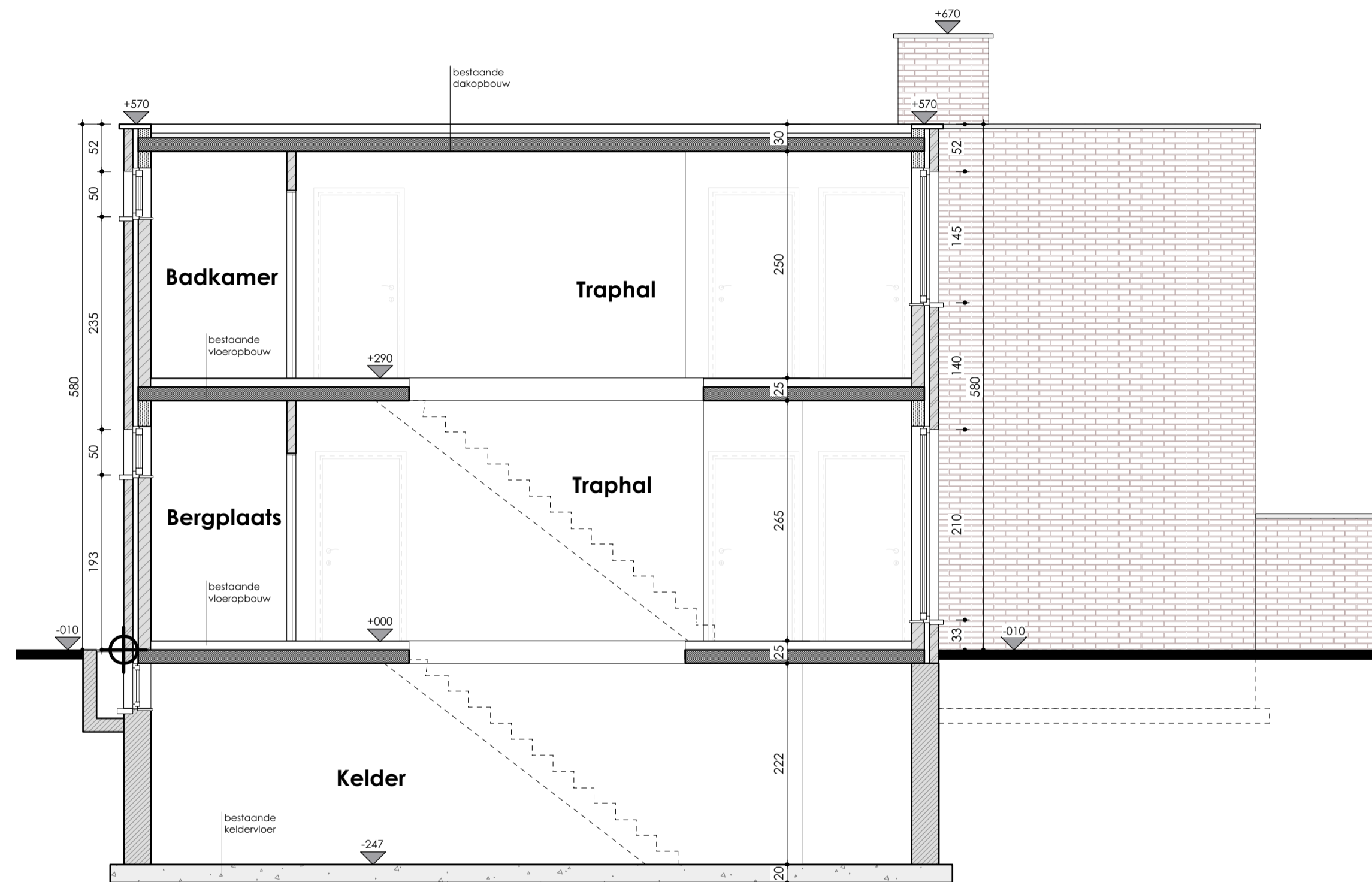
Doorsnede AA -Vergunde toestand Schaal: 1:50
