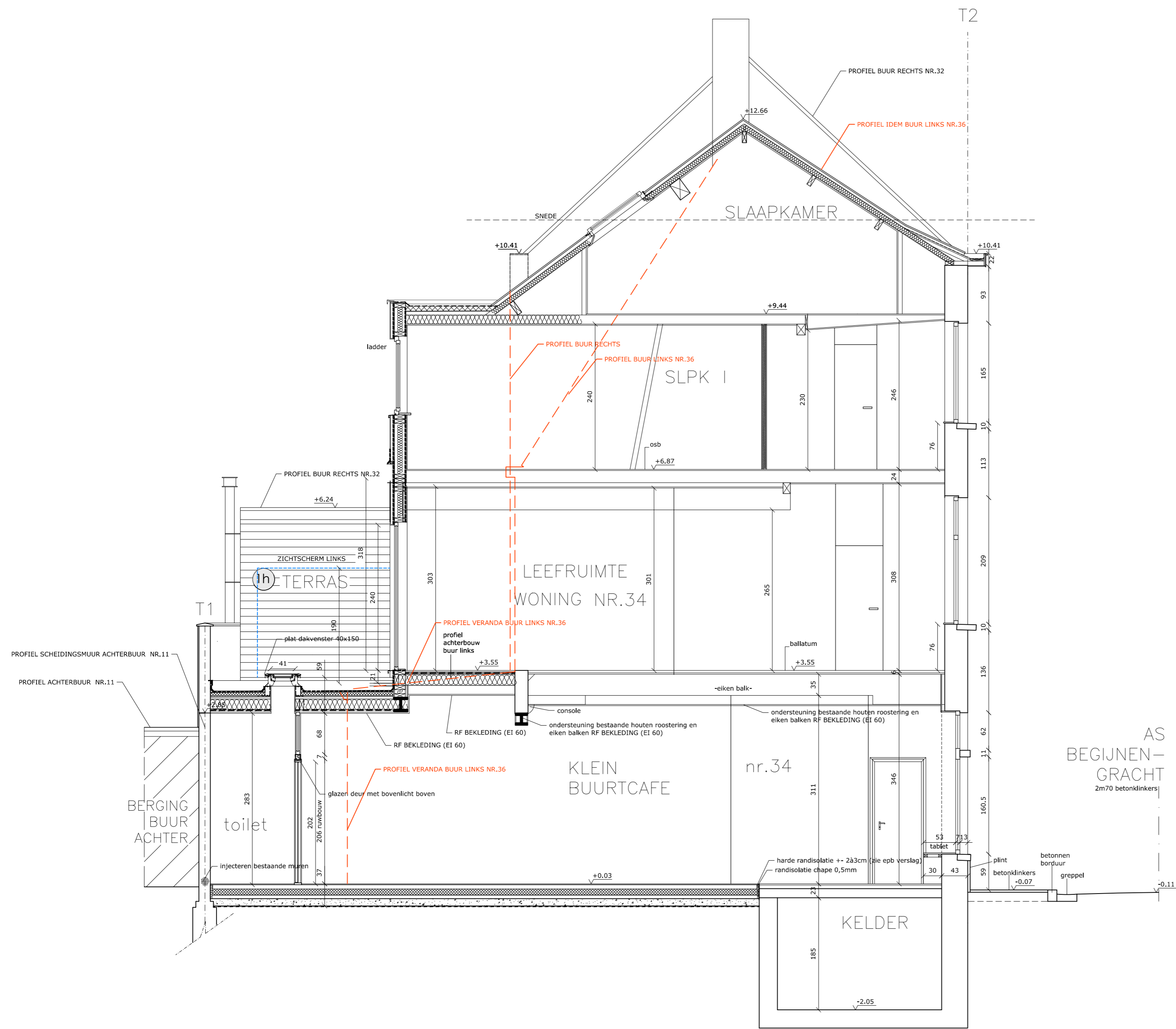
DOORSNEDE AA' / TERREINPROFIEL T1 - T2
