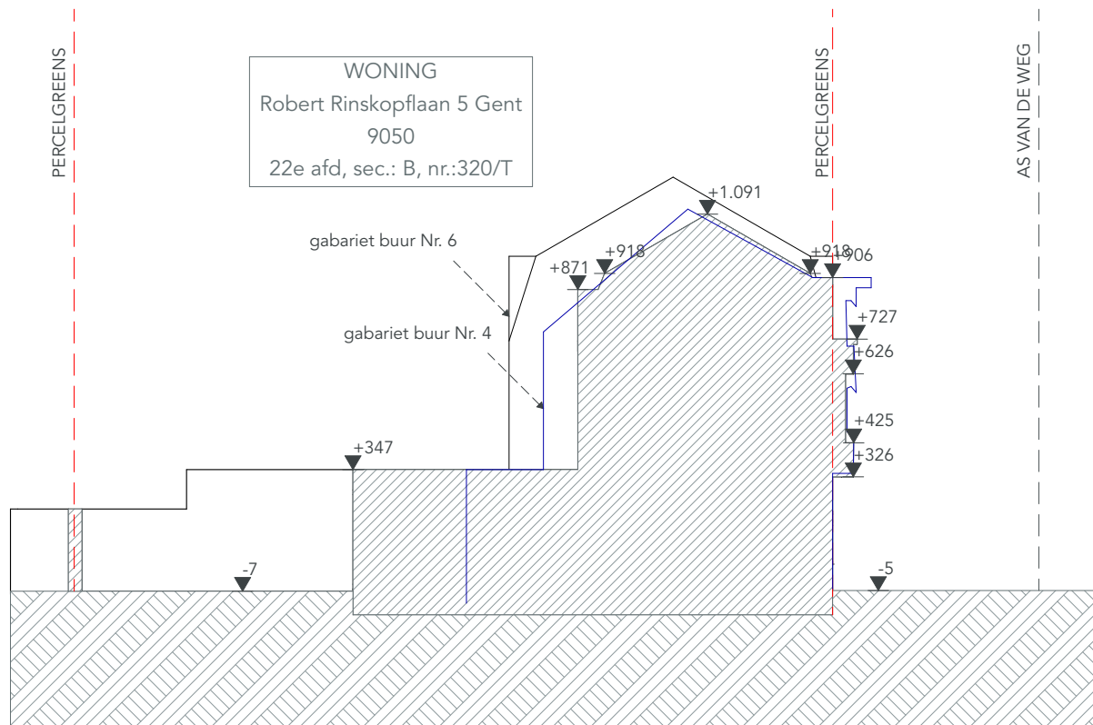
0 1 2 3 4 NT Terreinprofiel
