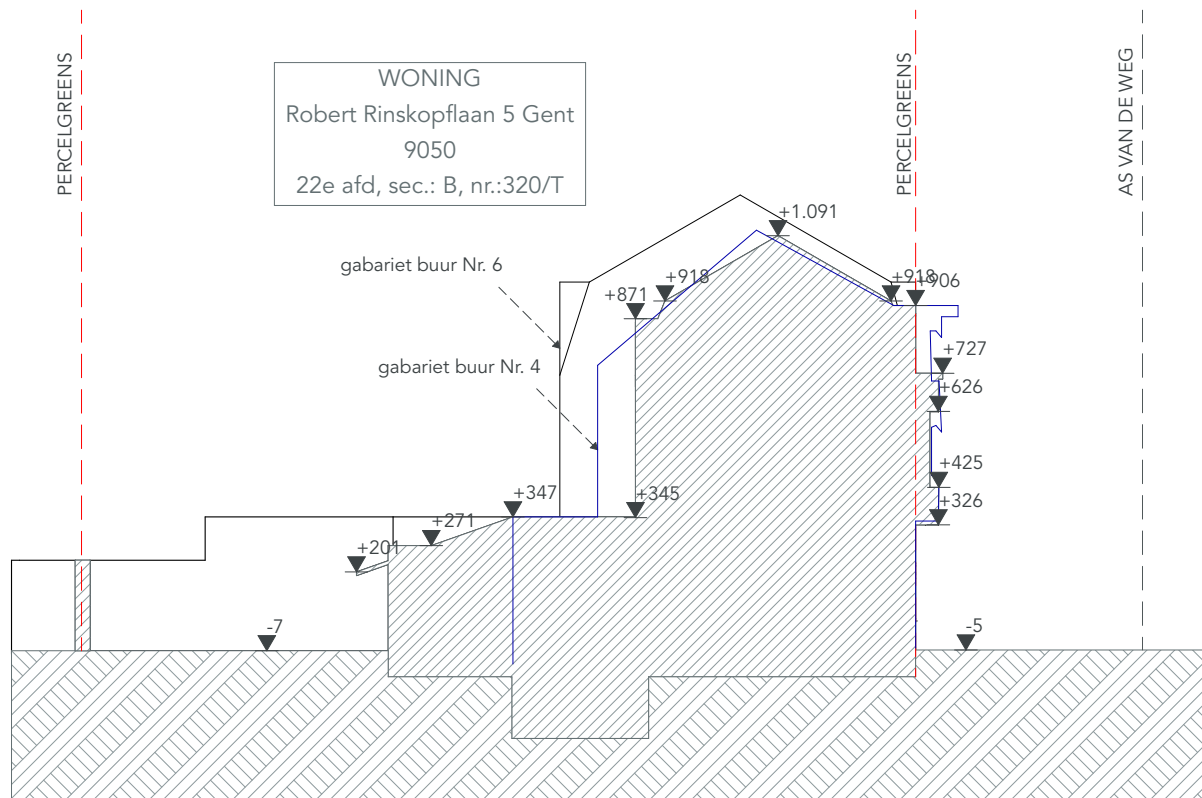
0 1 2 3 4 BT Terreinprofiel
