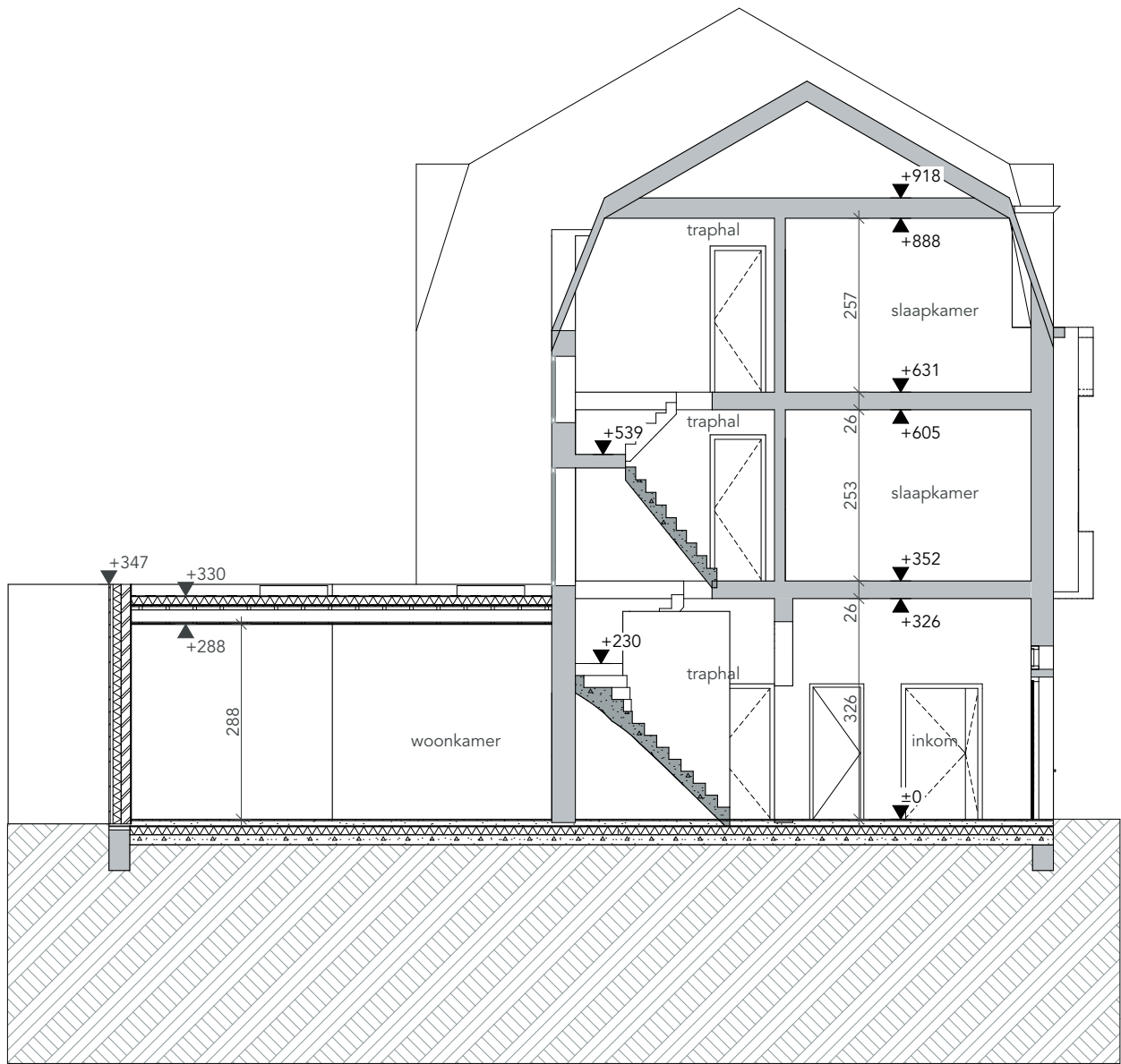
NT Doorsnede B-B
