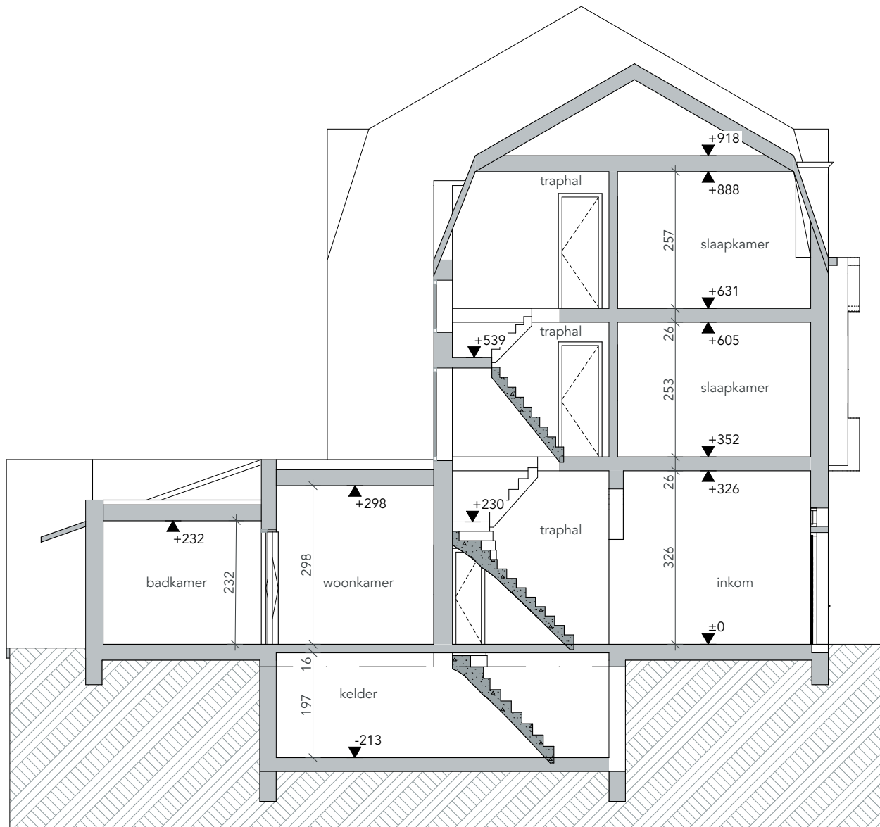
0 1 2 3 4 BT Doorsnede B-B
