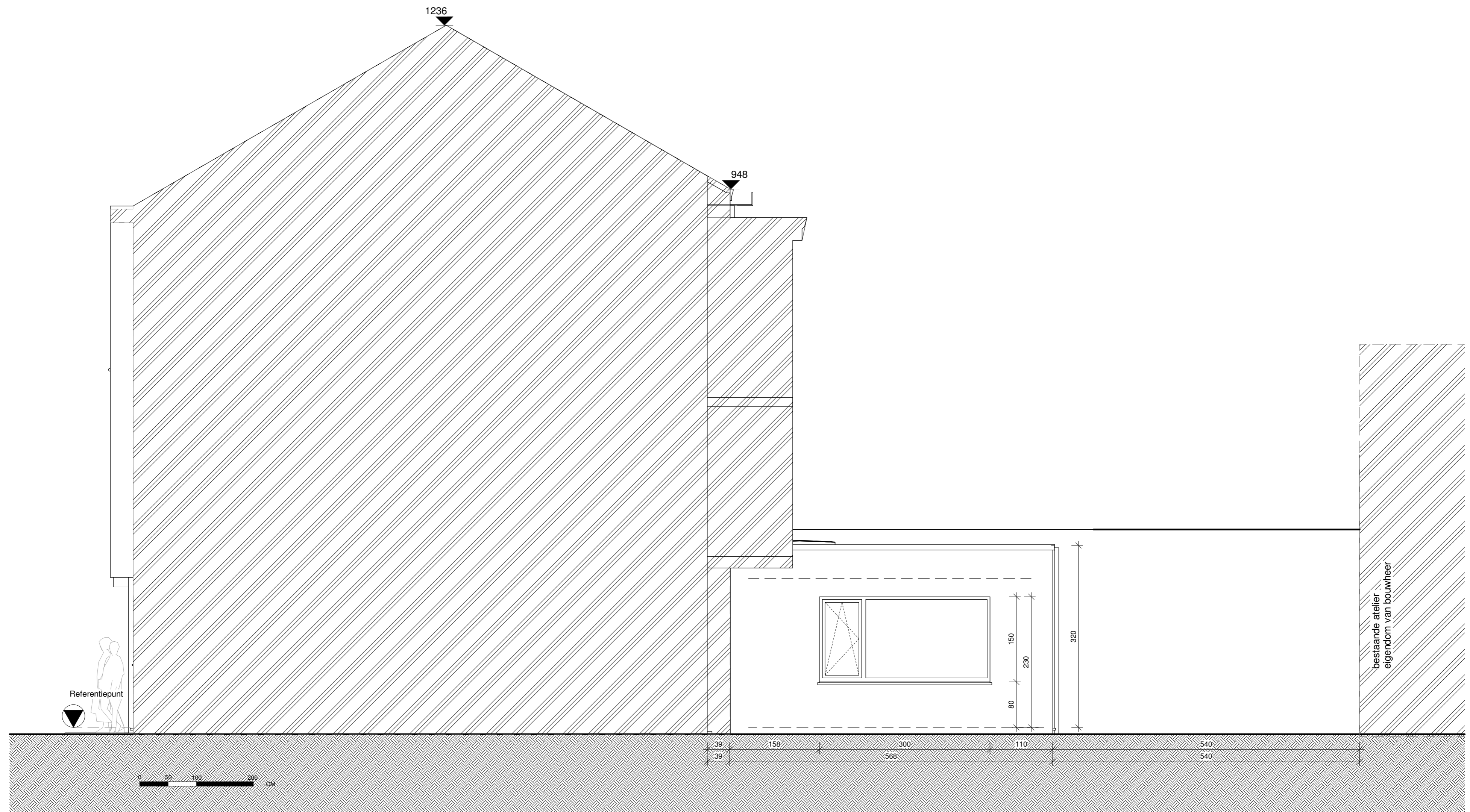
1 04_RECHTERGEVEL_nieuwe toestand 1 : 50
