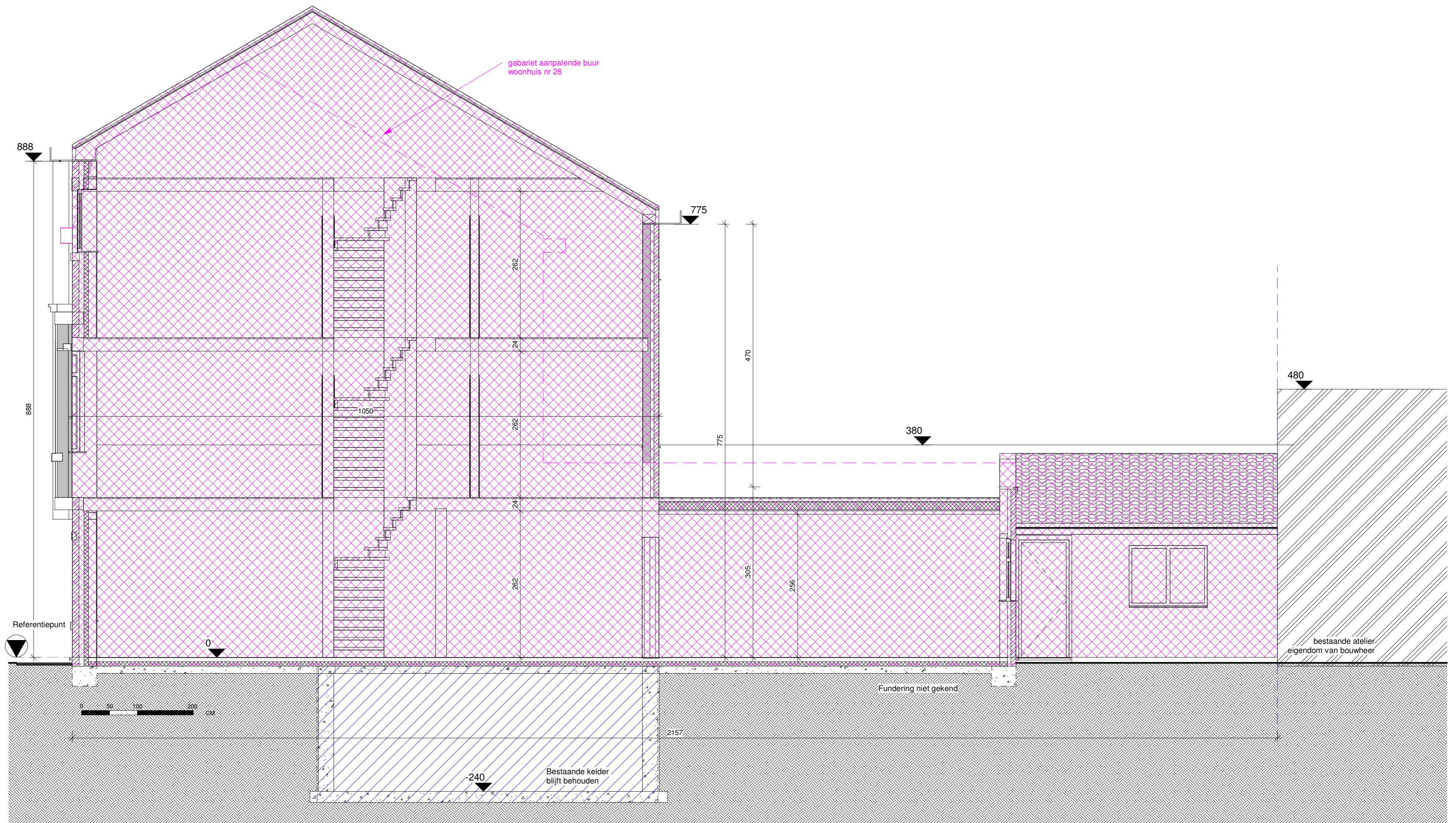
1 01_DOORSNEDE_bestaande toestand_TE SLOPEN 1 : 50
