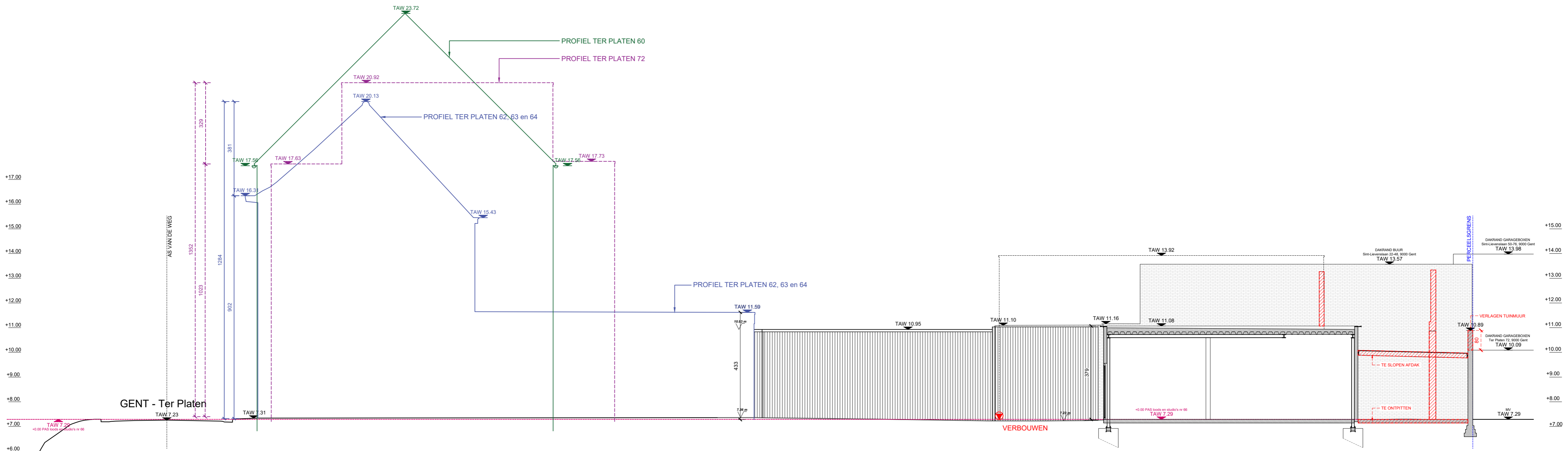
DOORSNEDE AA 0 100 200 300 400 cm 500 cm SCHAAL 1/100 BESTAANDE TOESTAND
