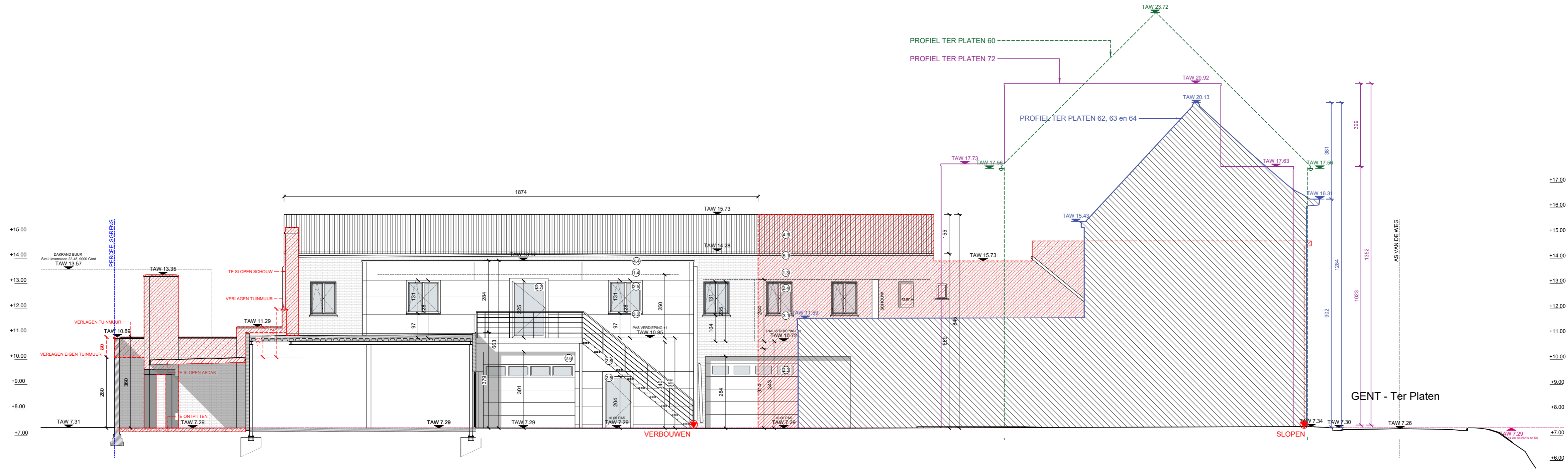
DOORSNED E AA '' 0 100 200 300 400 cm 500 cm SCHAAL 1/100 BESTAANDE TOESTAND
