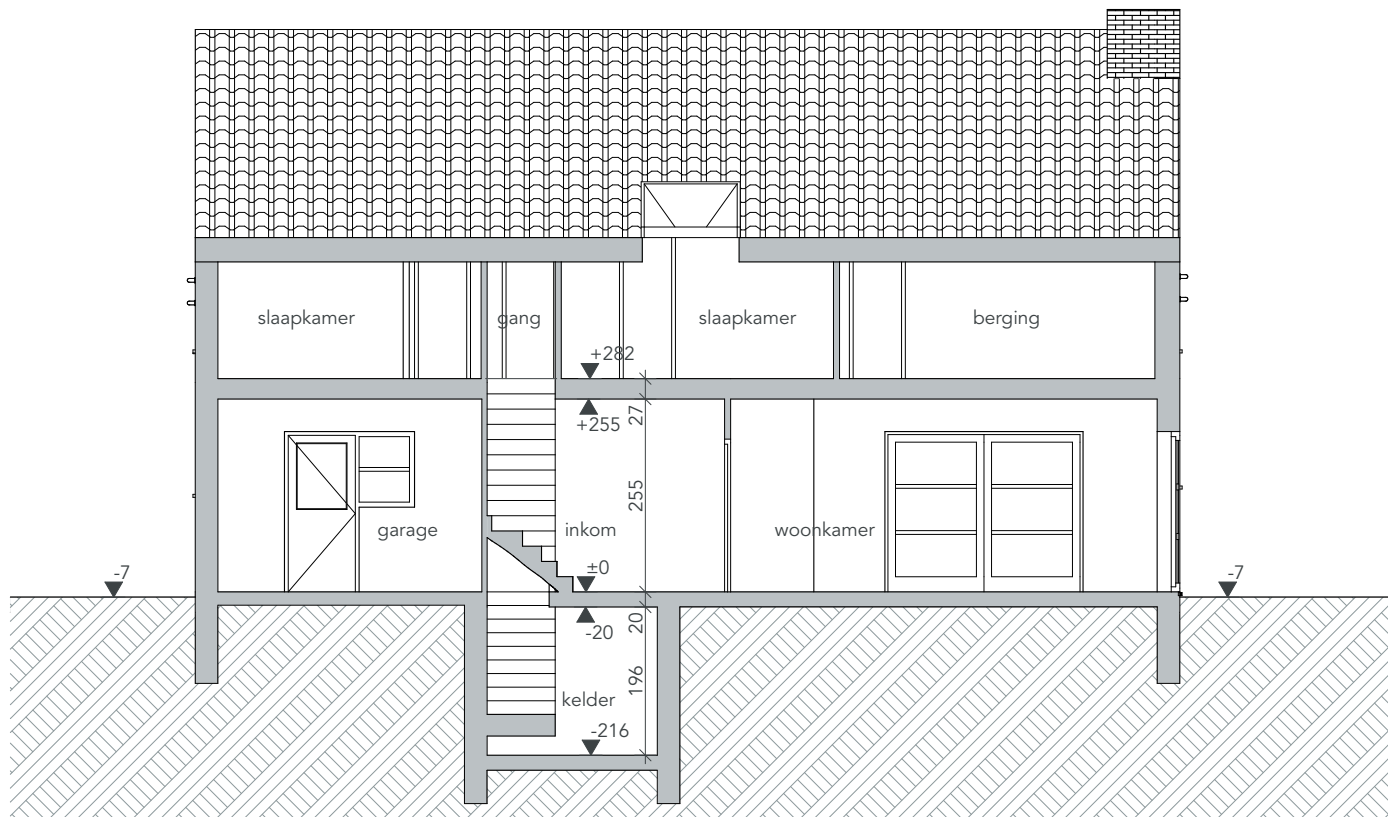
BT Doorsnede A-A
