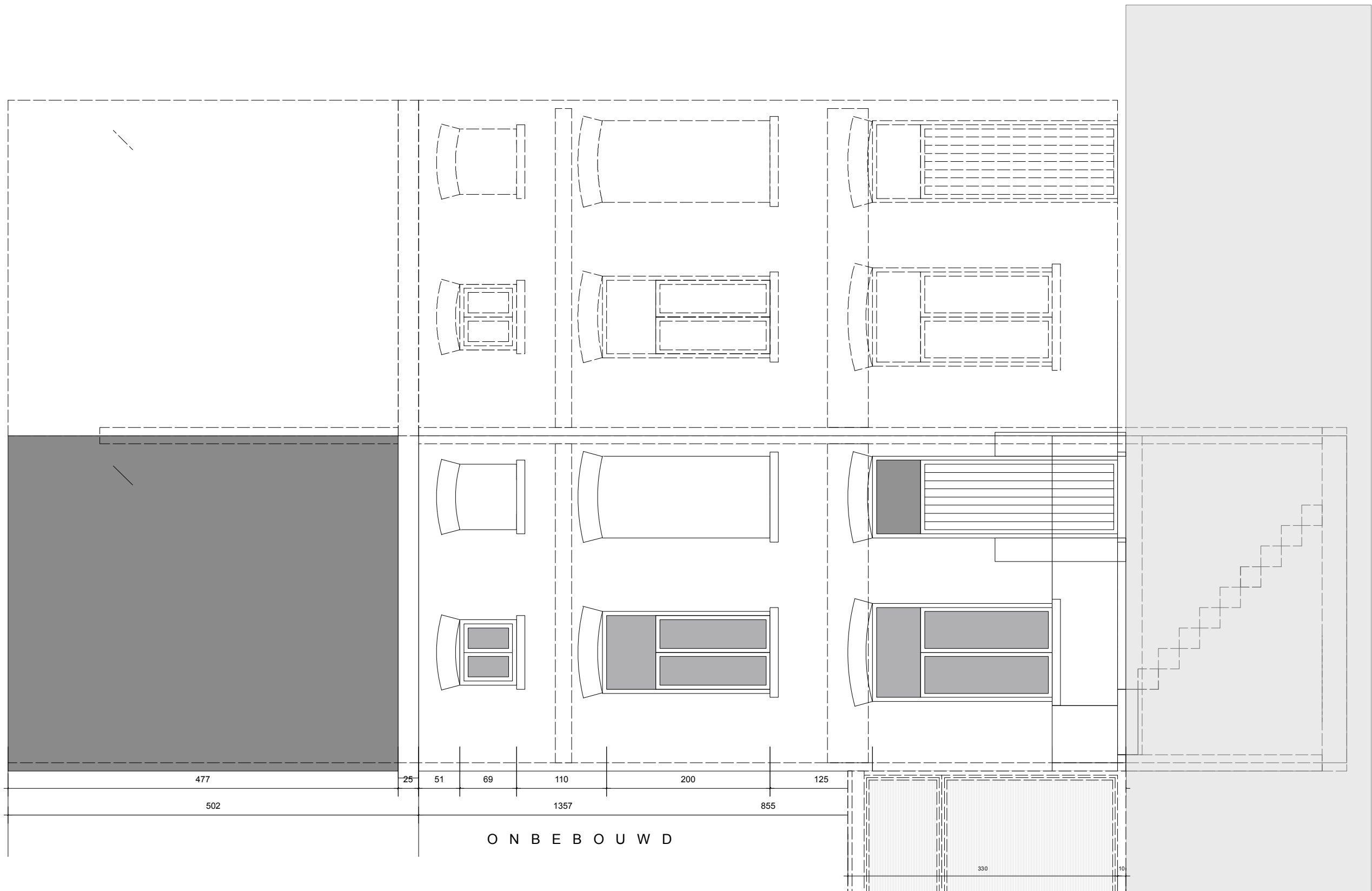
BA_VERBOUWEN RIJWONING_G_B_1_STRAATGEVEL SCHAAAL 1/50
