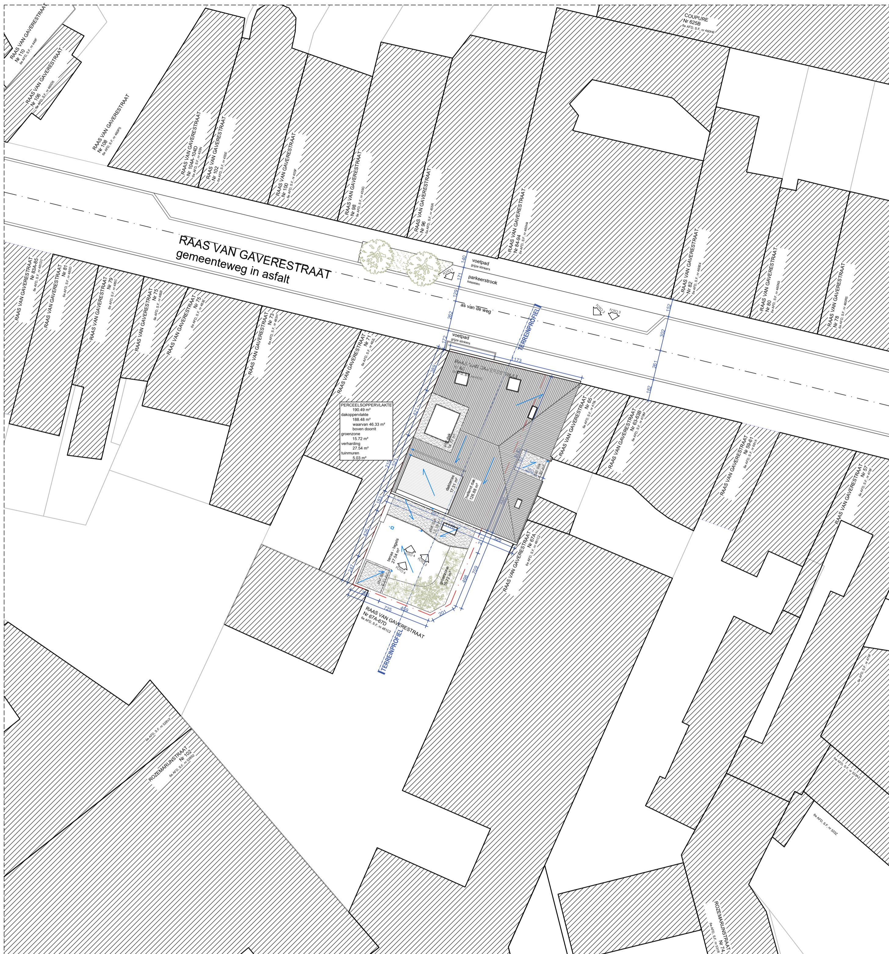
INPLANTINGSPLAN vergunde toestand - schaal 1/200
