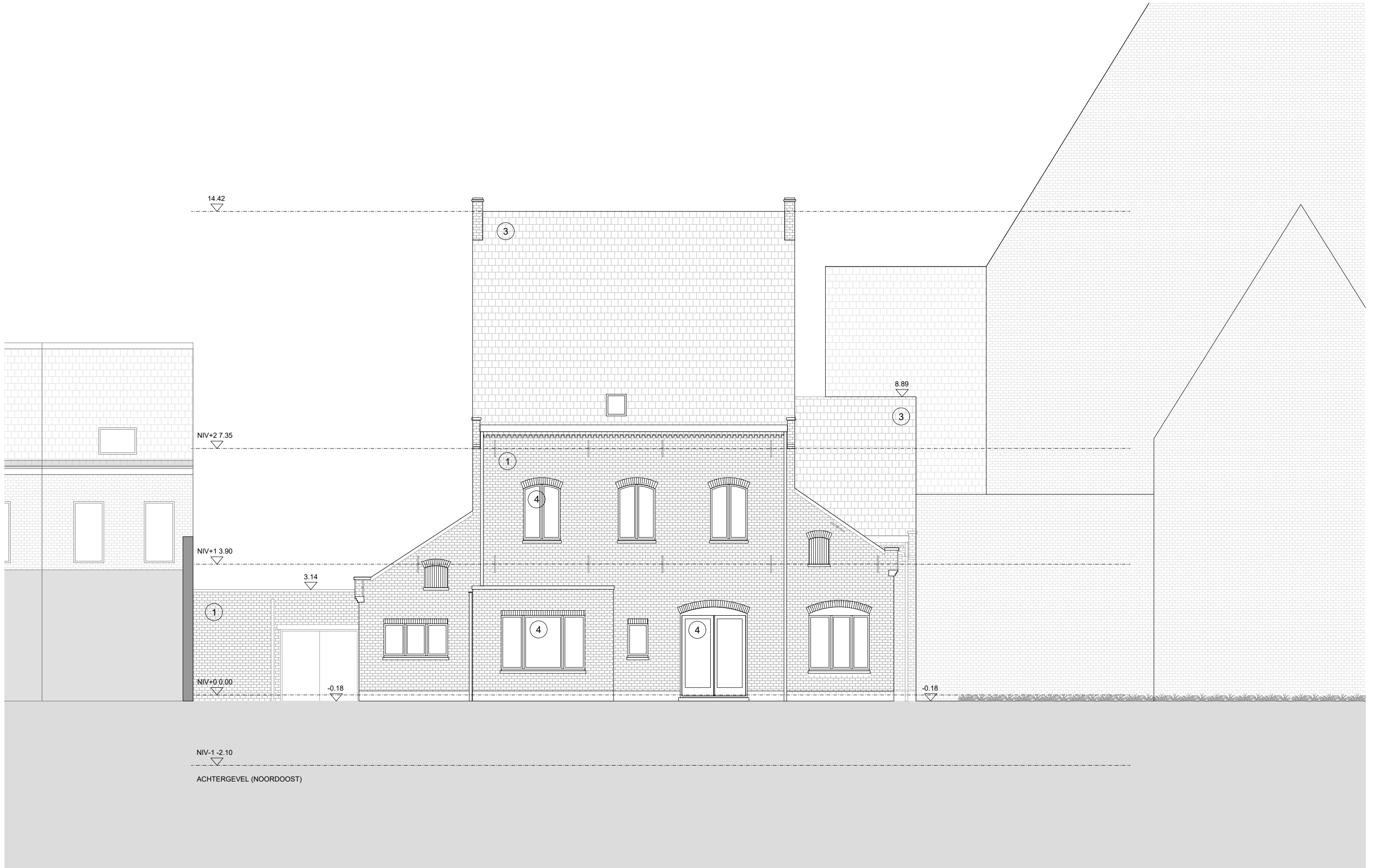
KEIBERG 1 - GENTBRUGGE ACHTERGEVEL noordoost - bestaande toestand
