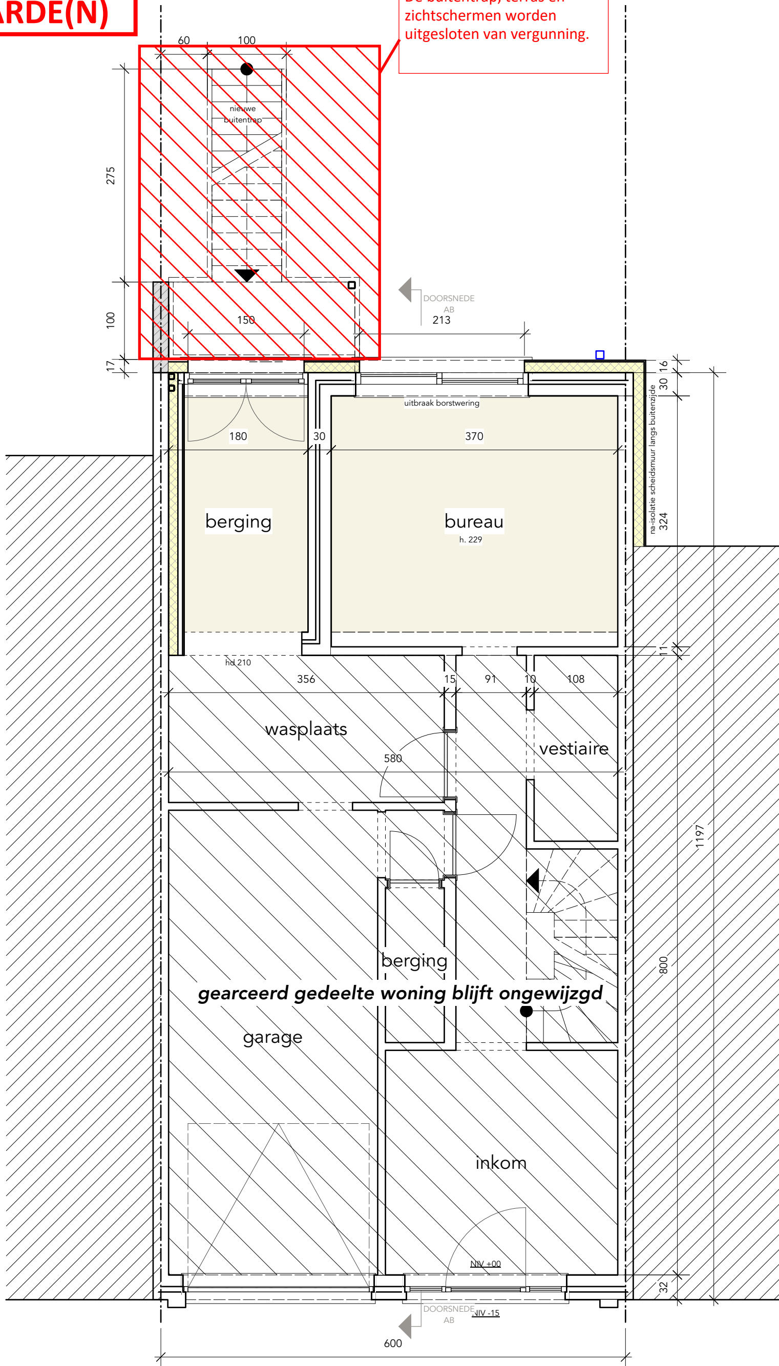
PLAN GELIJKVLOERS
