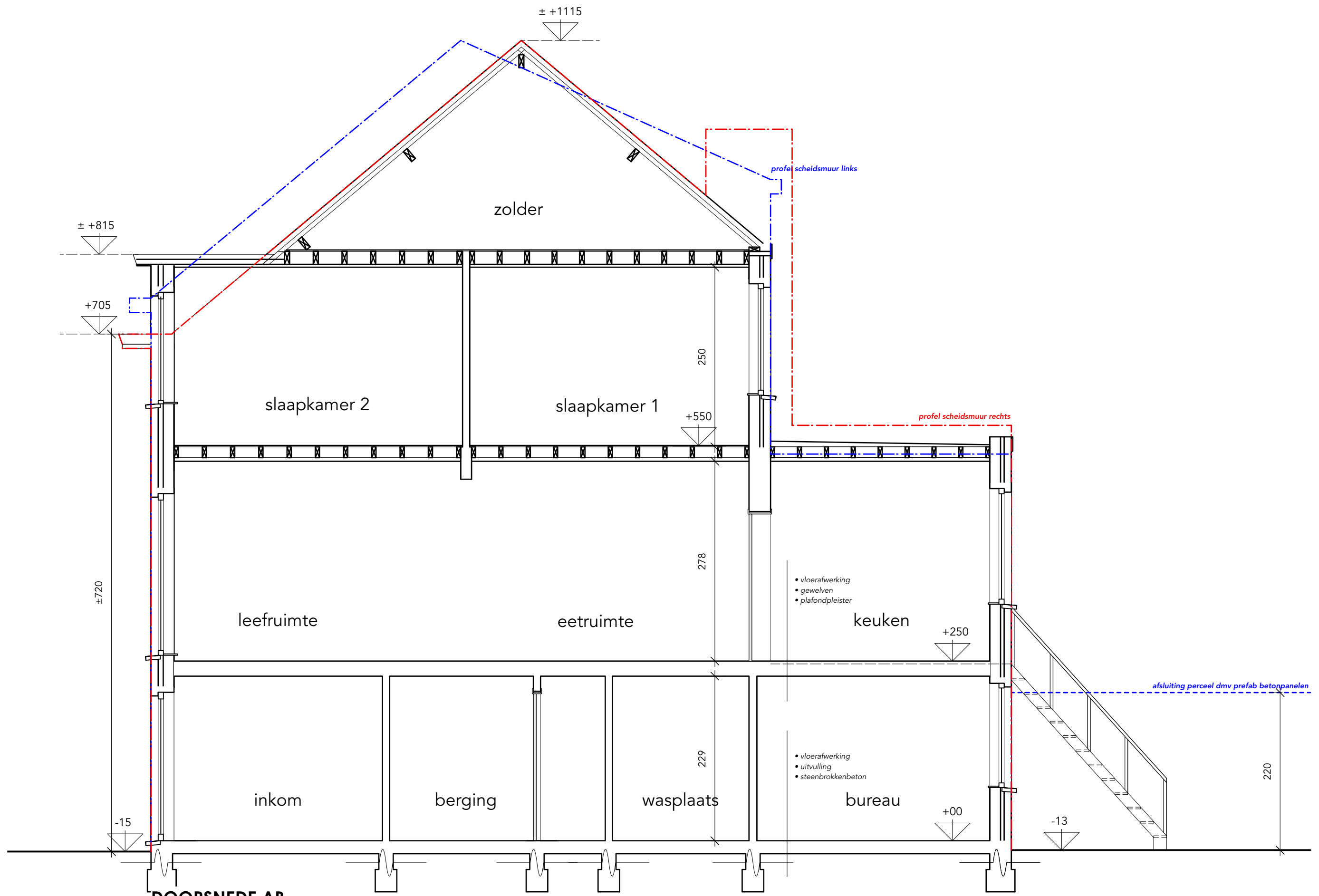
DOORSNEDE AB
