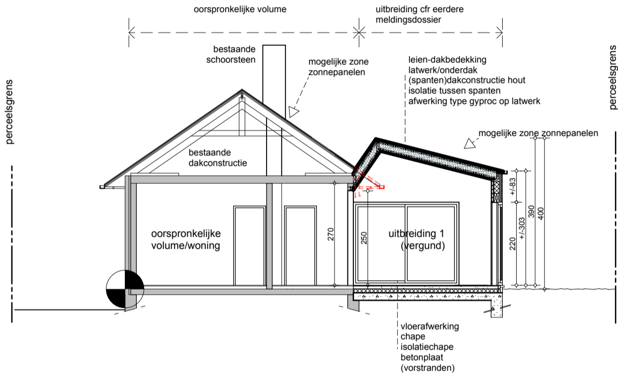
Basisschema doorsnede oorspronkelijk volume + uitbreiding (cfr eerdere meldingsdossier)
