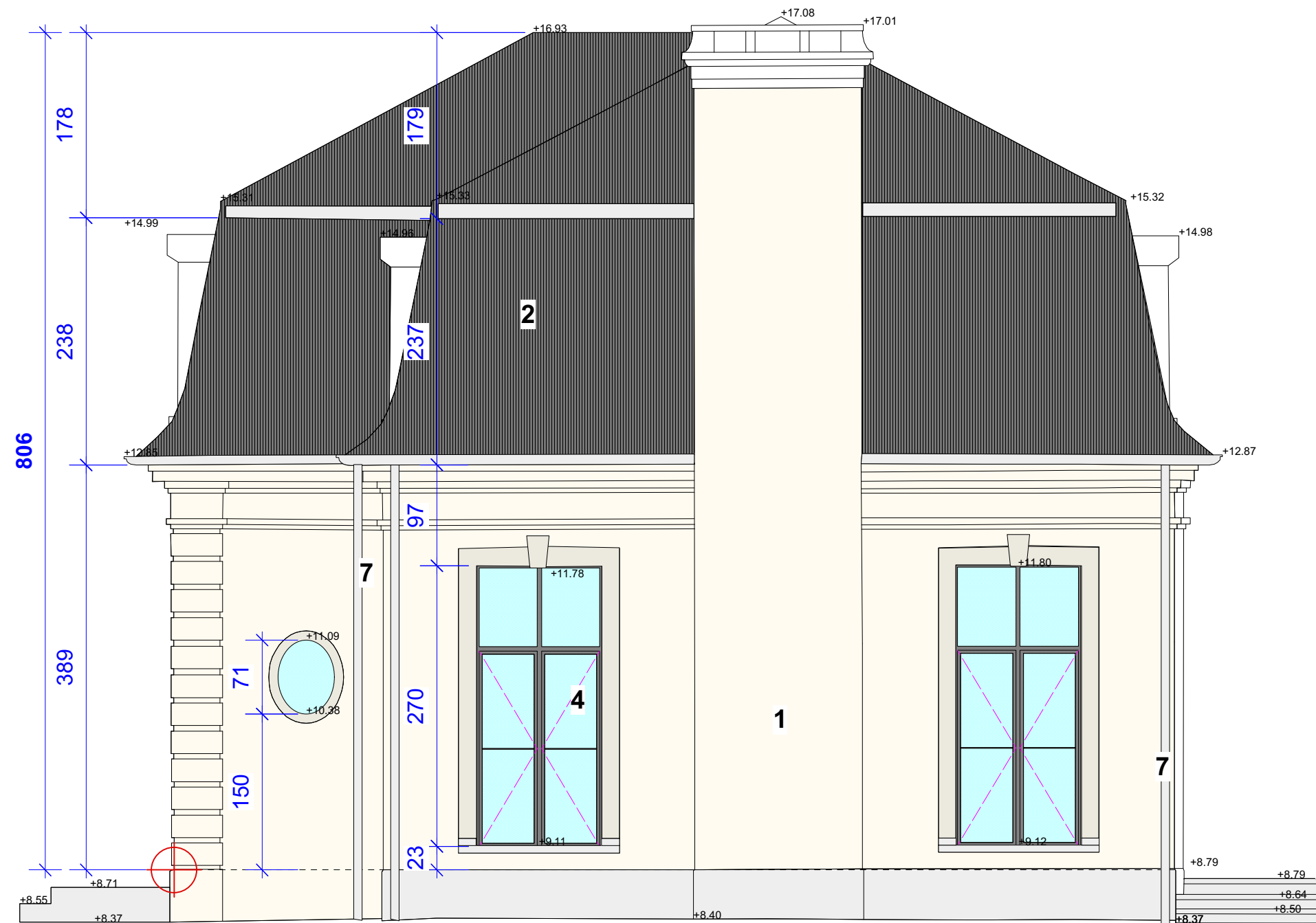
WONING - ZIJGEVEL RECHTS nieuwe toestand
