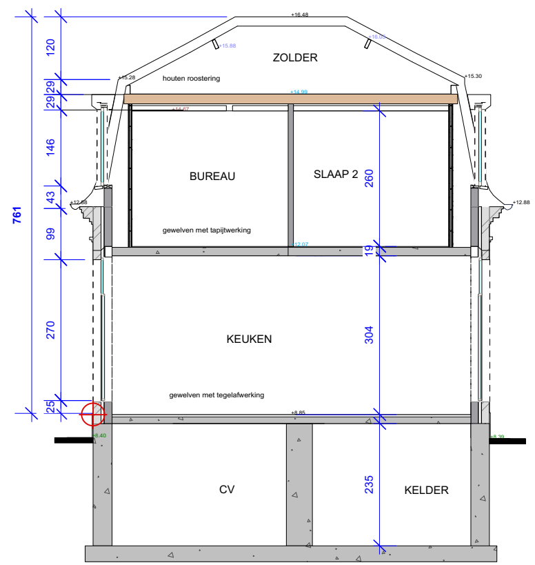
DOORSNEDE 2'-2'
