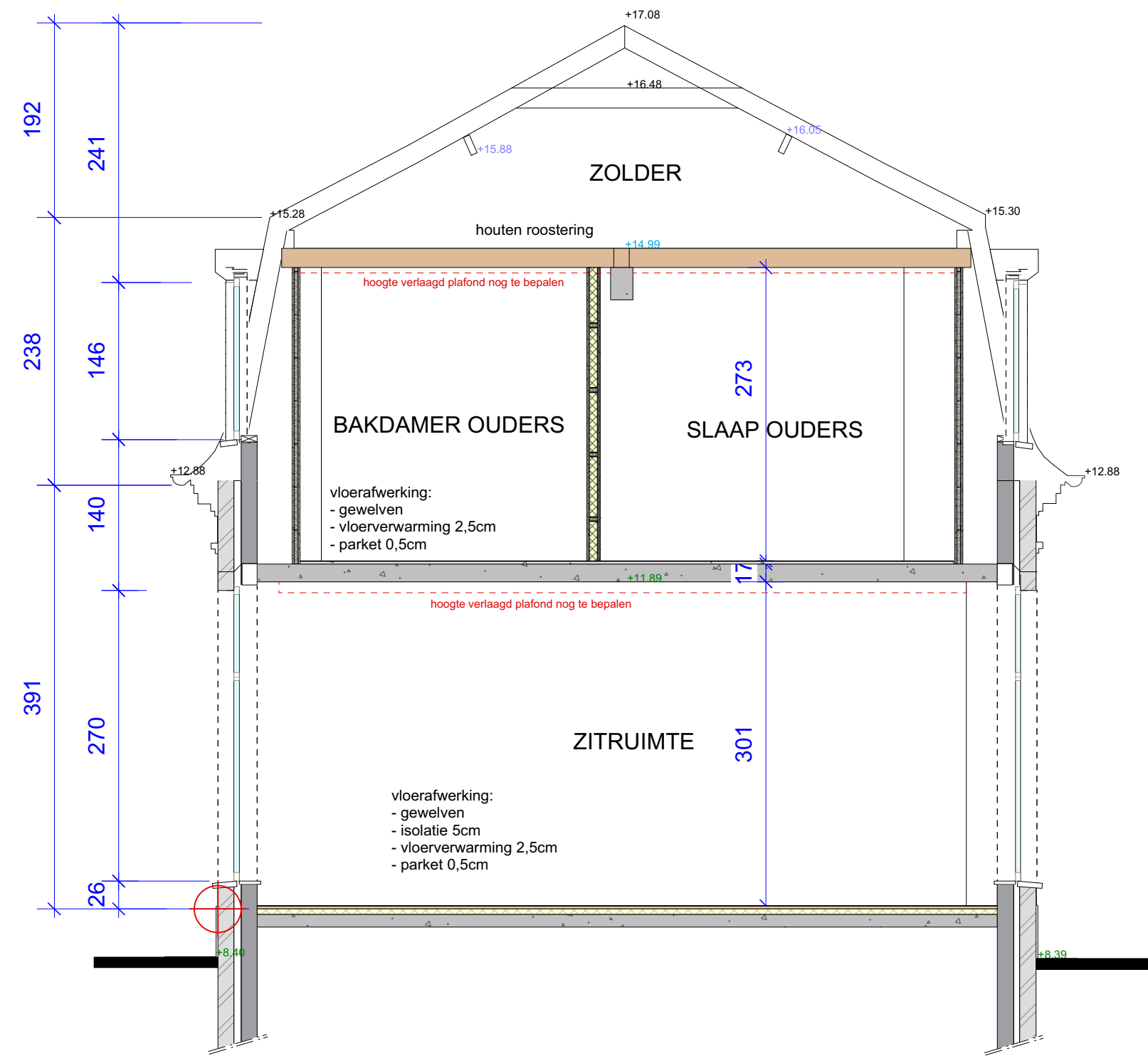
DOORSNEDE 1-1
