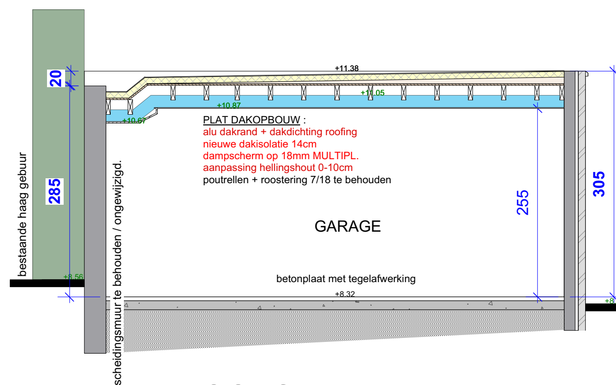
DOORSNEDE 4-4
