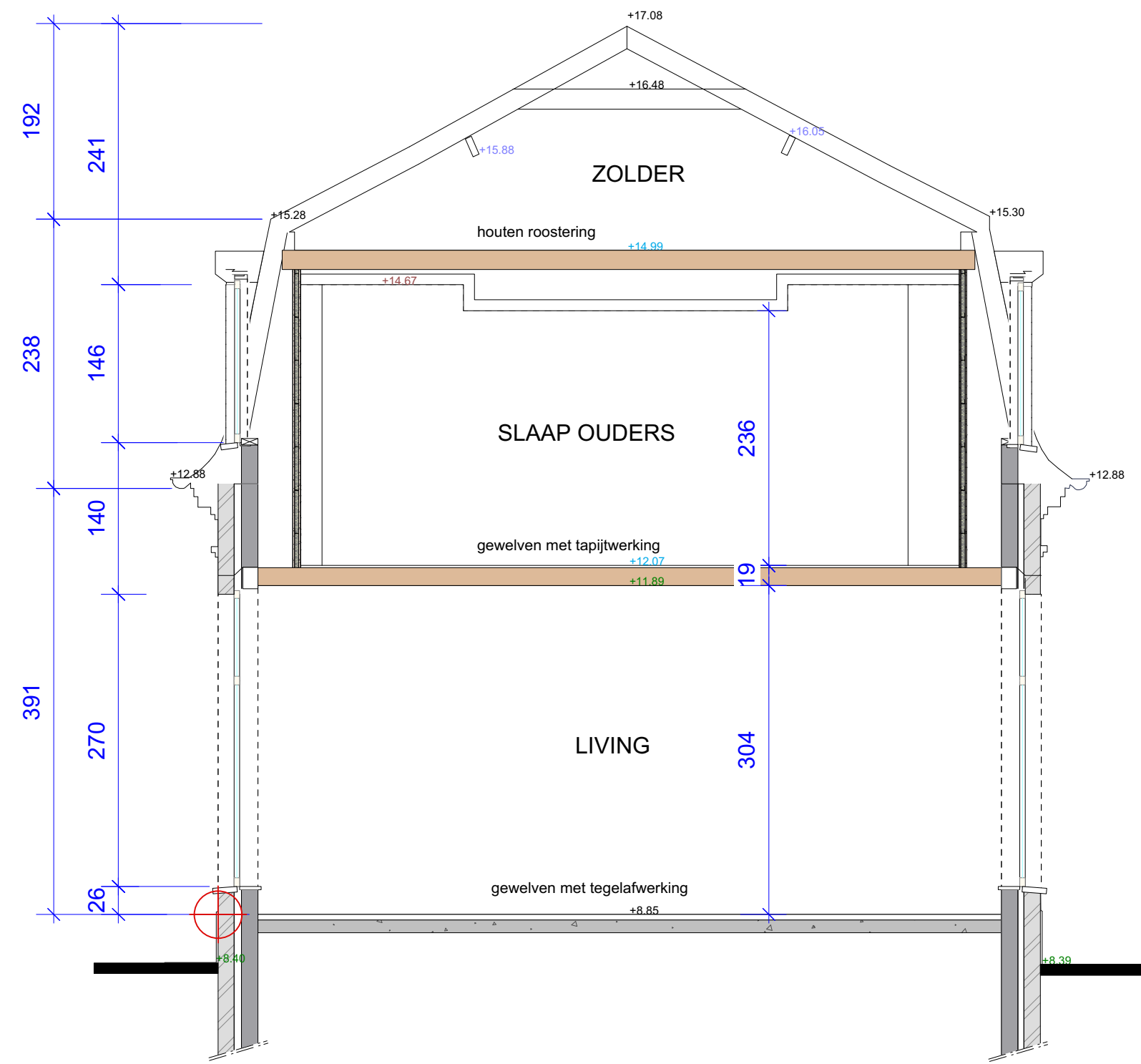
DOORSNEDE 1-1
