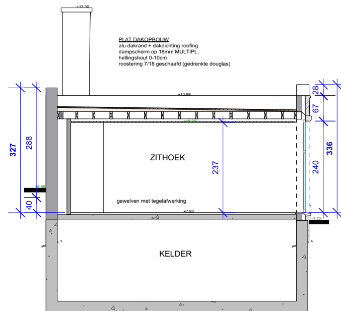
DOORSNEDE 6-6
