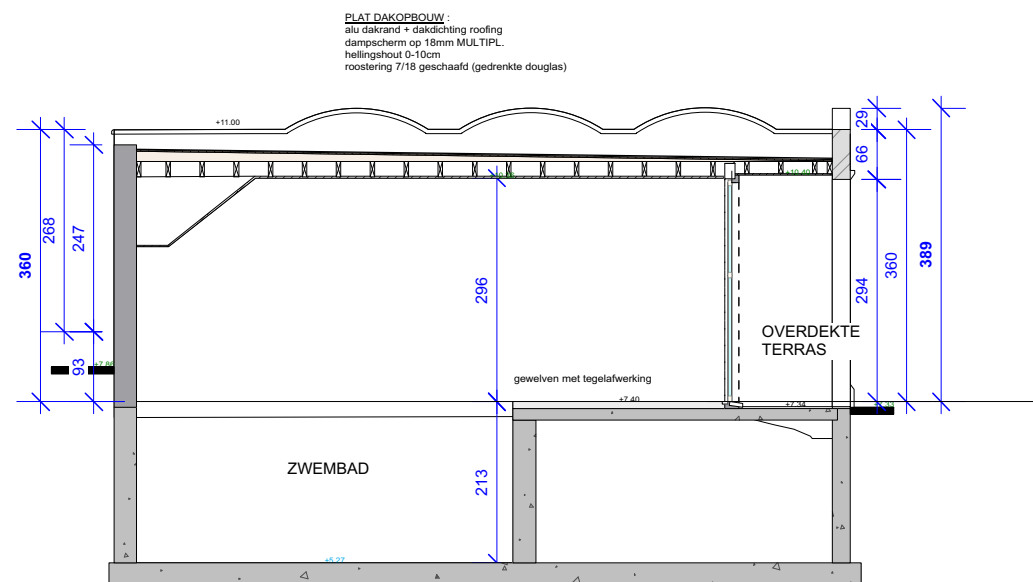
DOORSNEDE 7-7
