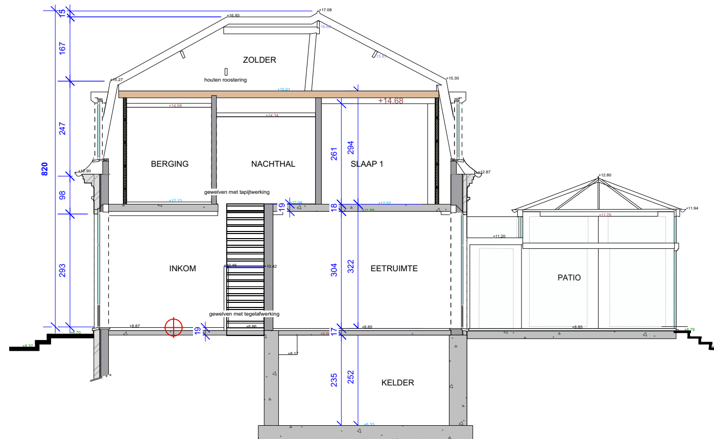
DOORSNEDE 2-2
