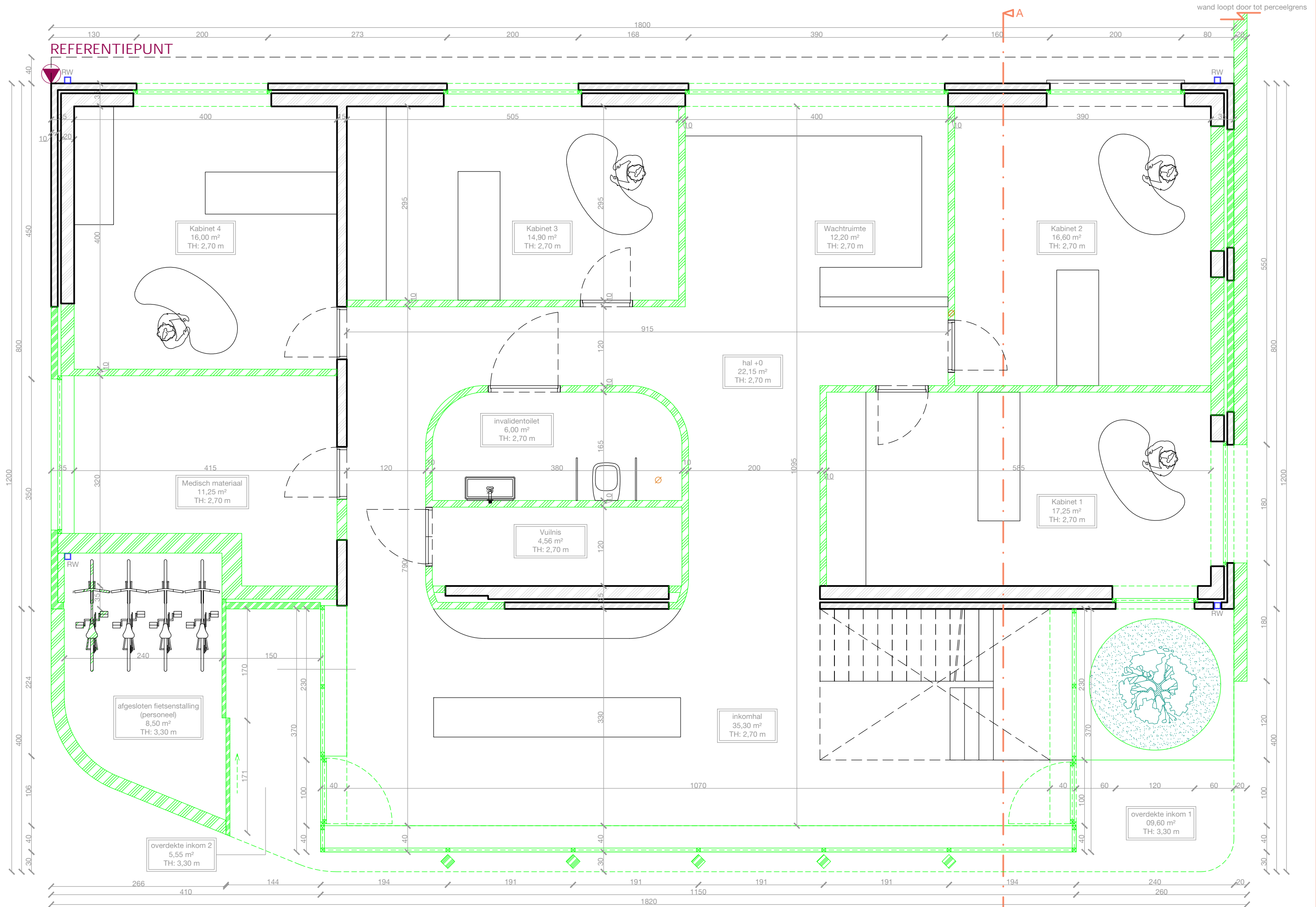
GRONDPLAN GELIJKVLOERS- nieuwe situatie 1:50
