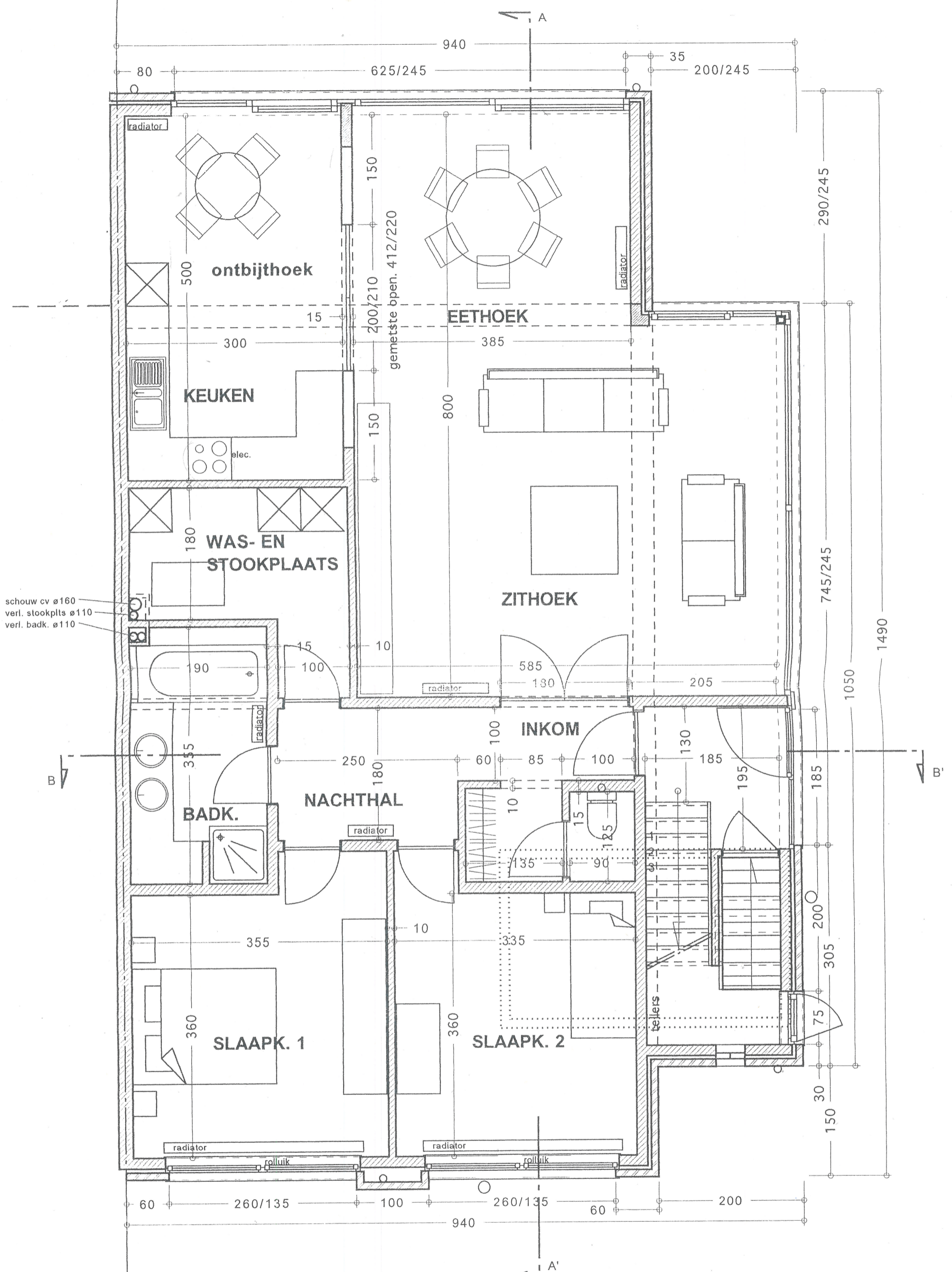
GRONDPLAN Bestaande Toestand niv. 0.00
