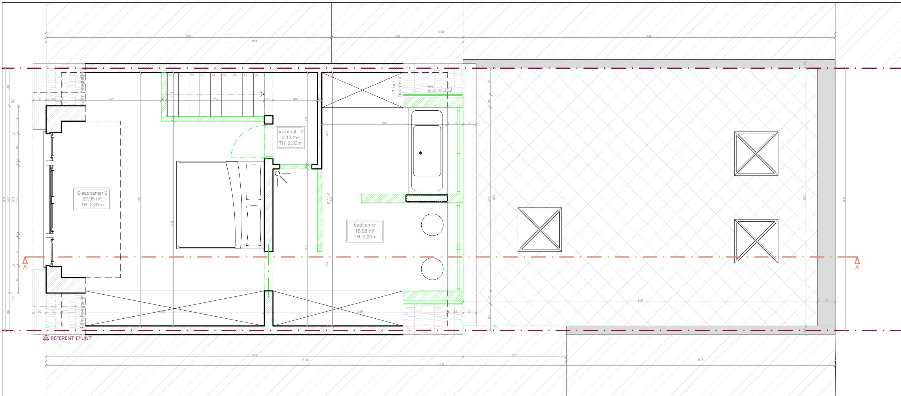
Grondplan verdieping +2- nieuwe situatie
