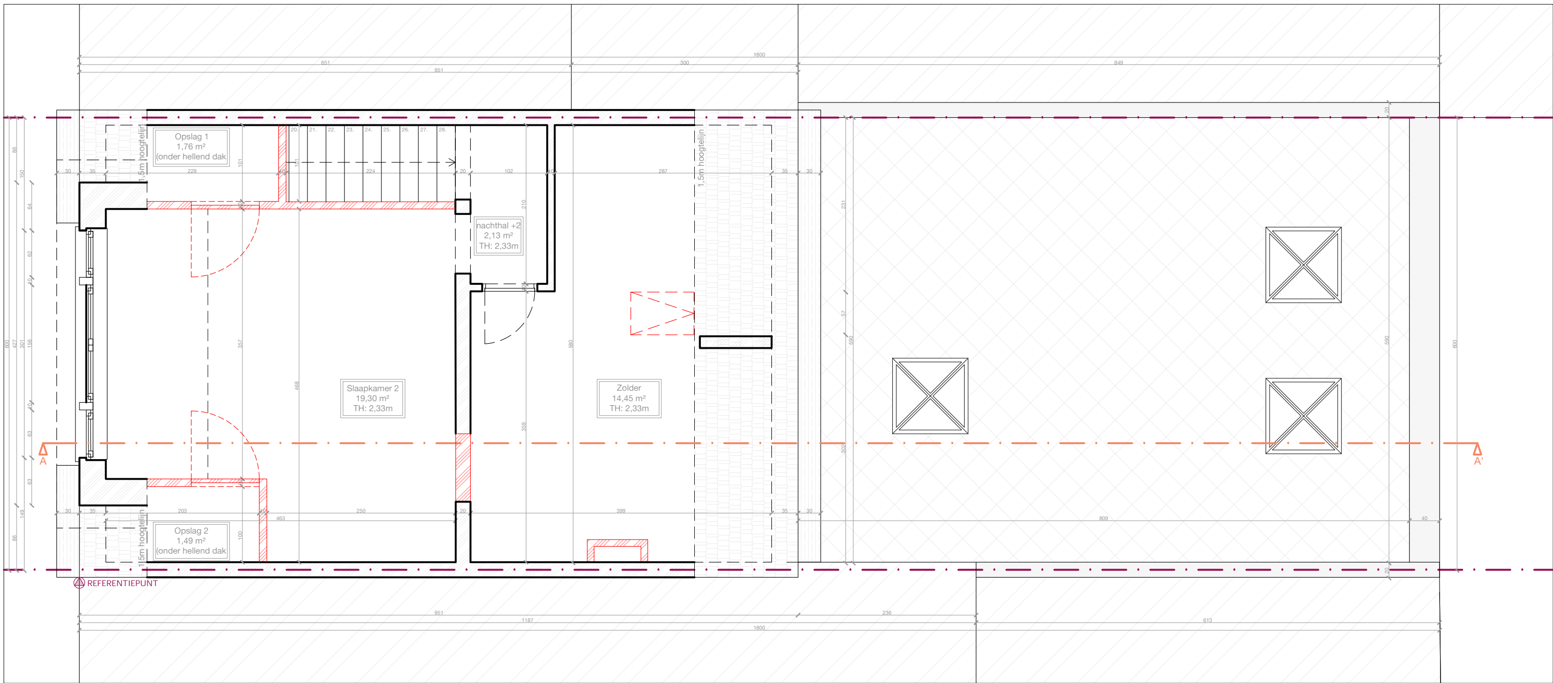
Grondplan verdieping +2- bestaande situatie
