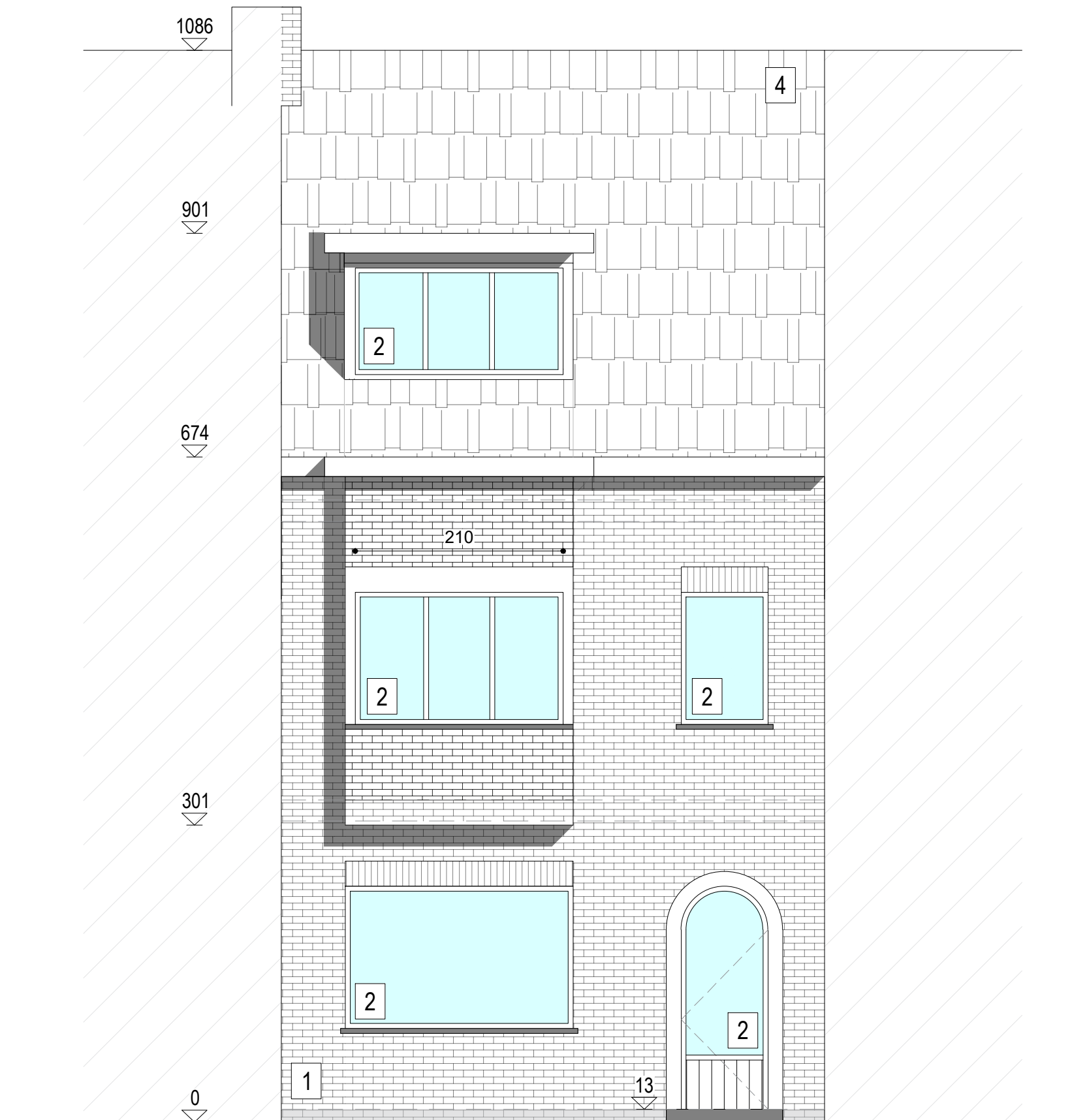
VOORGEVEL Bestaande toestand Schaal 1/50
