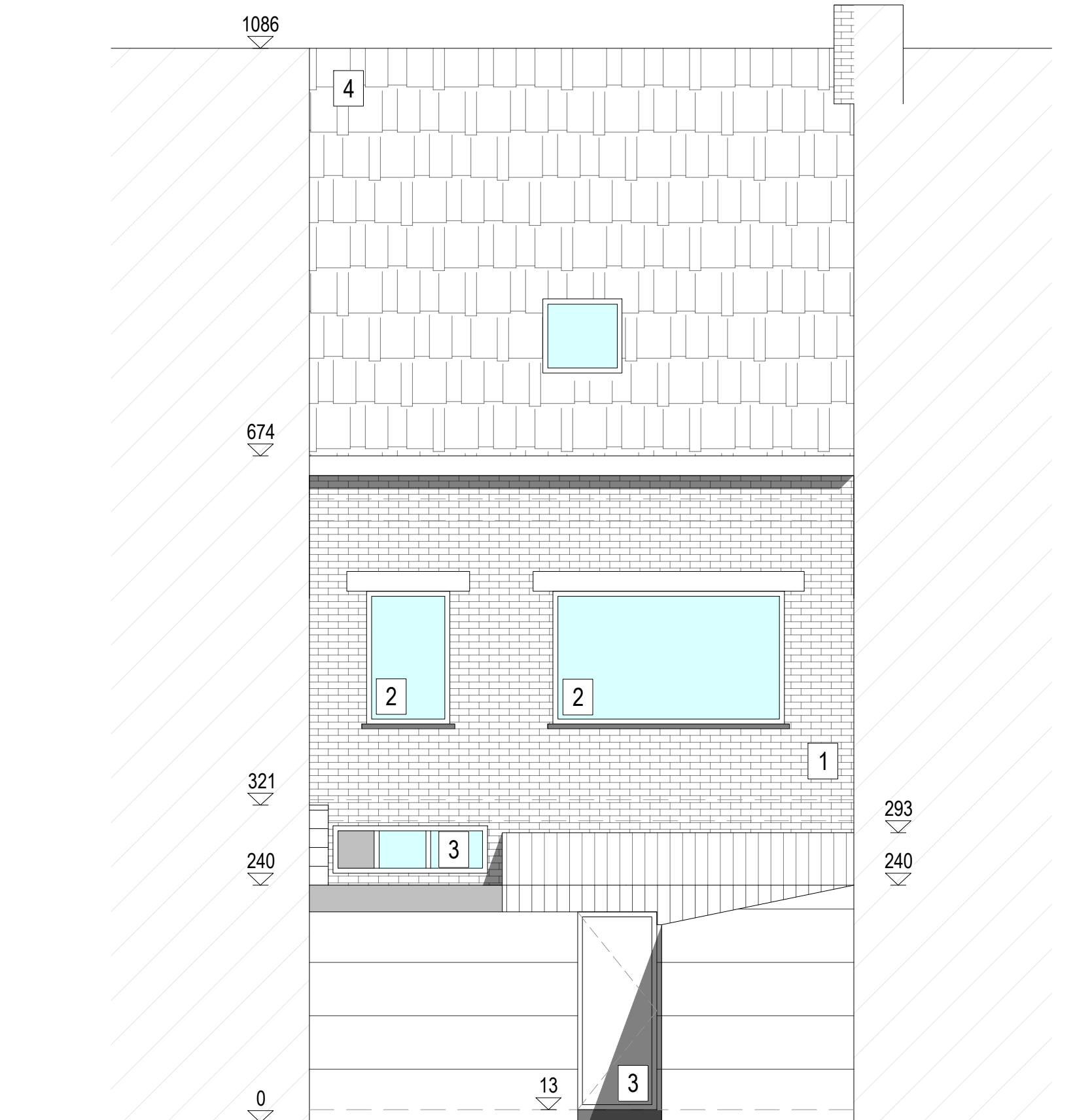
ACHTERGEVEL Bestaande toestand Schaal 1/50
