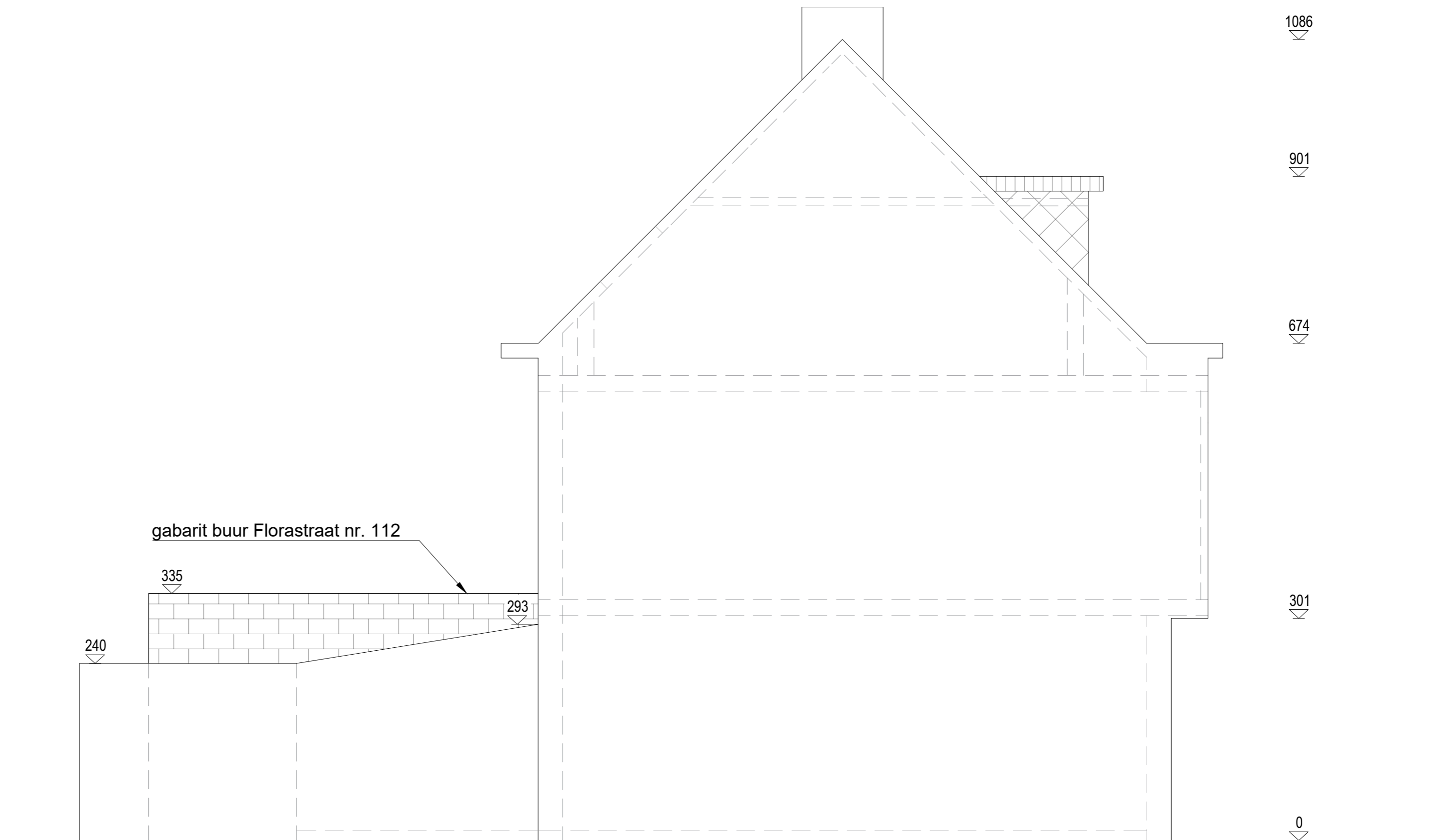
LINKER ZIJGEVEL Bestaande toestand Schaal 1/50
