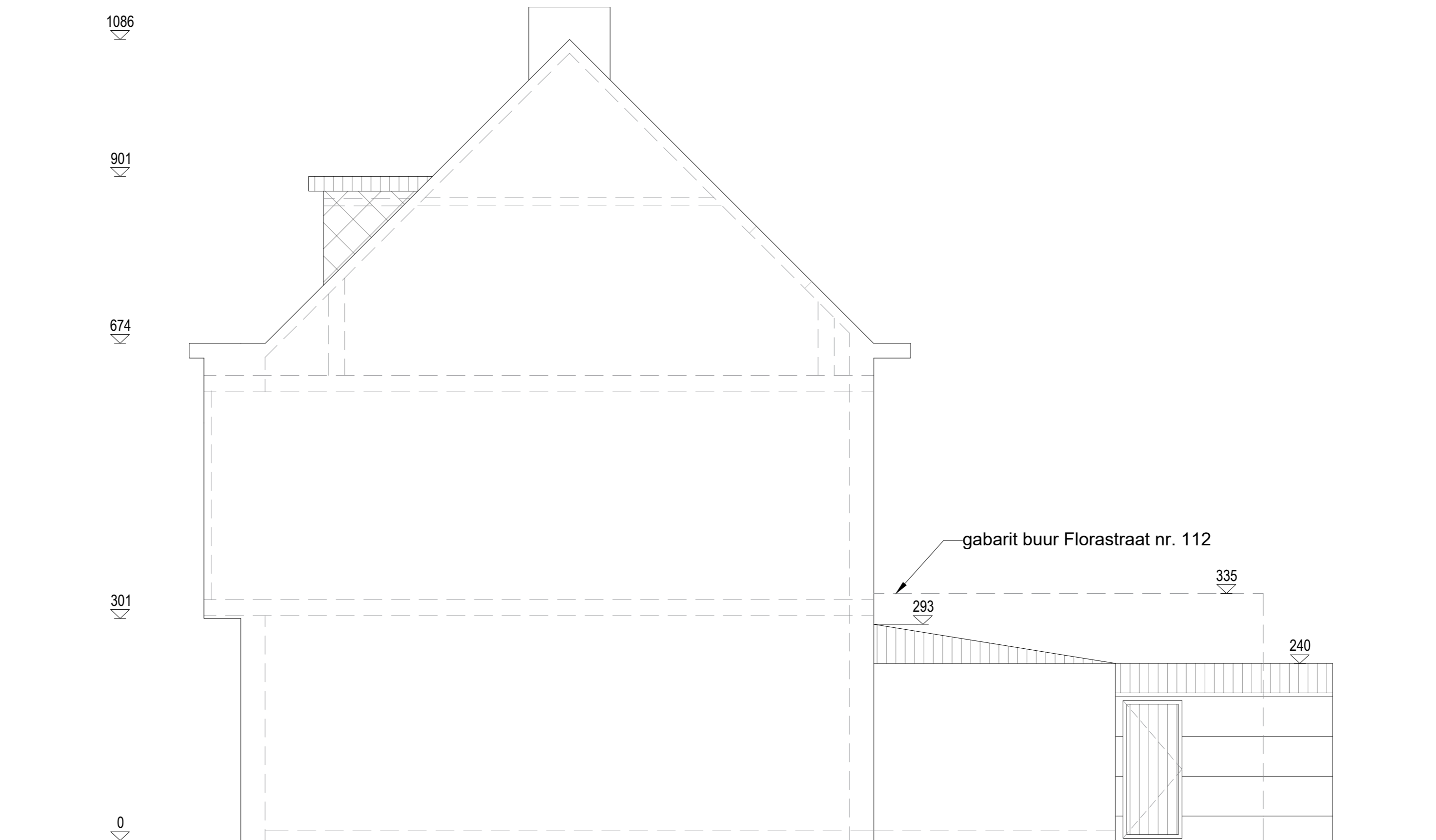
RECHTER ZIJGEVEL Bestaande toestand Schaal 1/50
