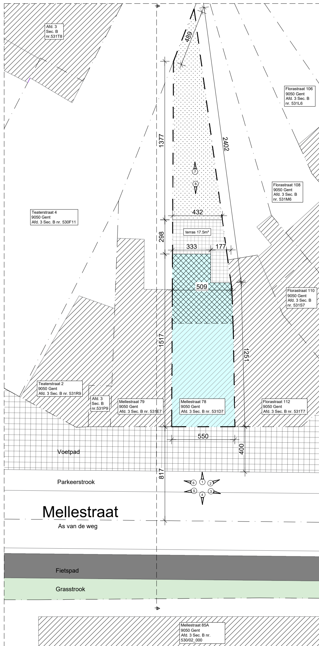
INPLANTING Bestaande toestand Schaal 1/200
