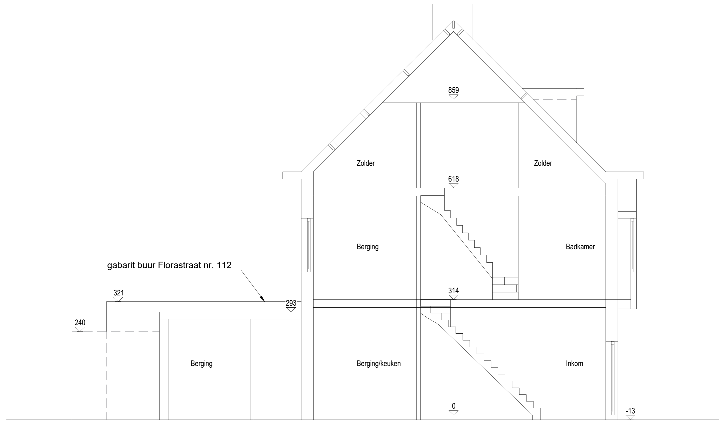
Snede AA' Bestaande toestand Schaal 1/50
