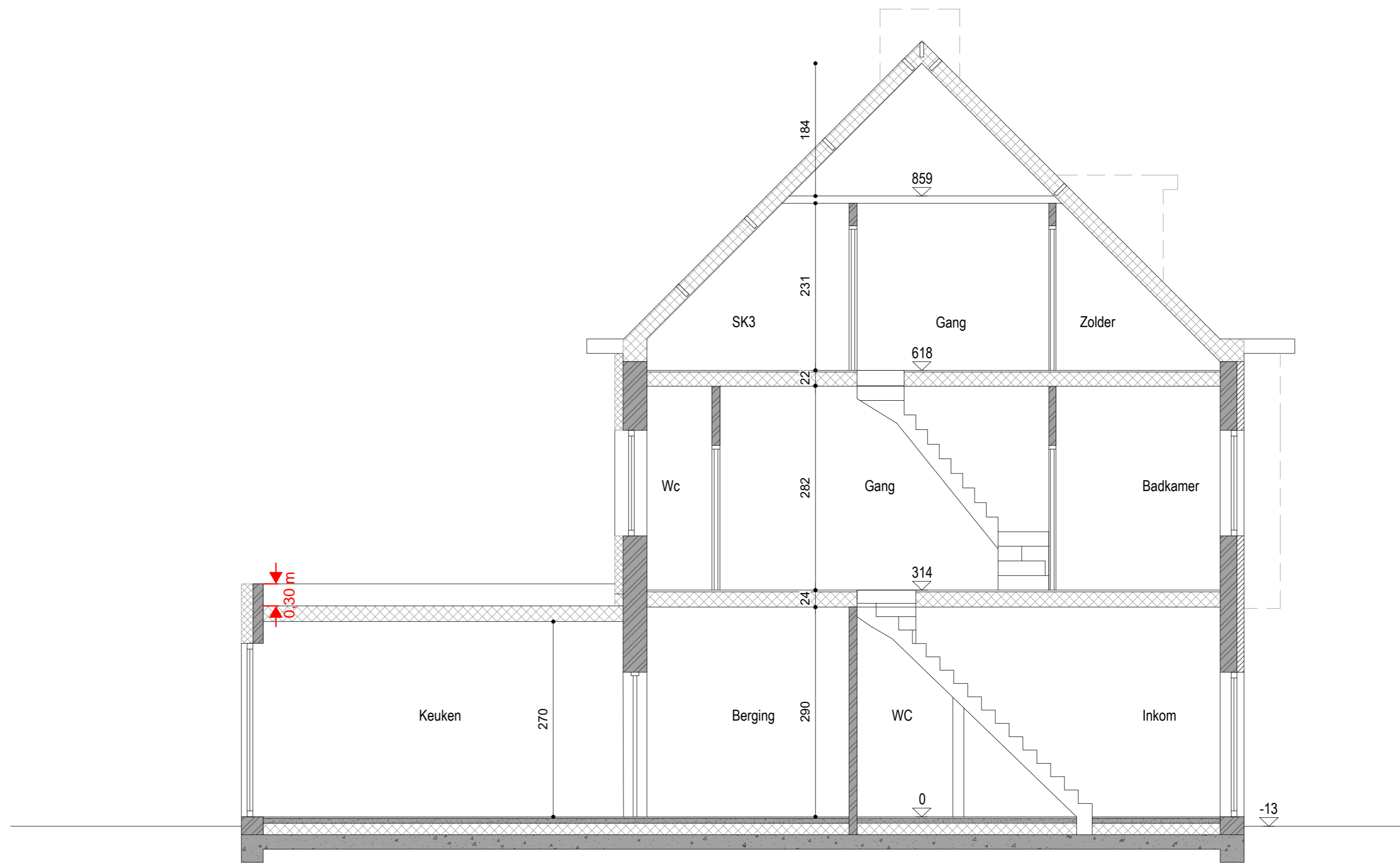
SNEDE AA' Nieuwe toestand Schaal 1/50
