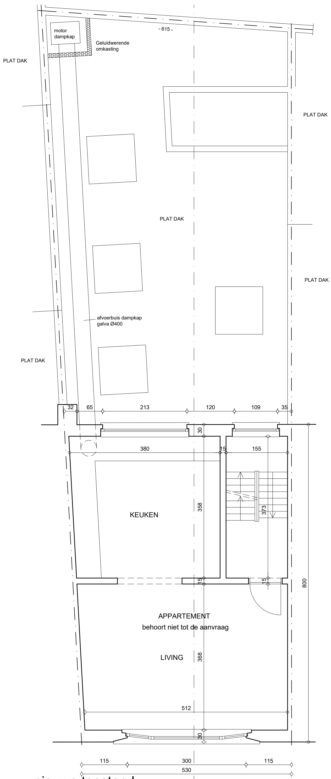
nieuwe toestand VERDIEPING 1 1:50
