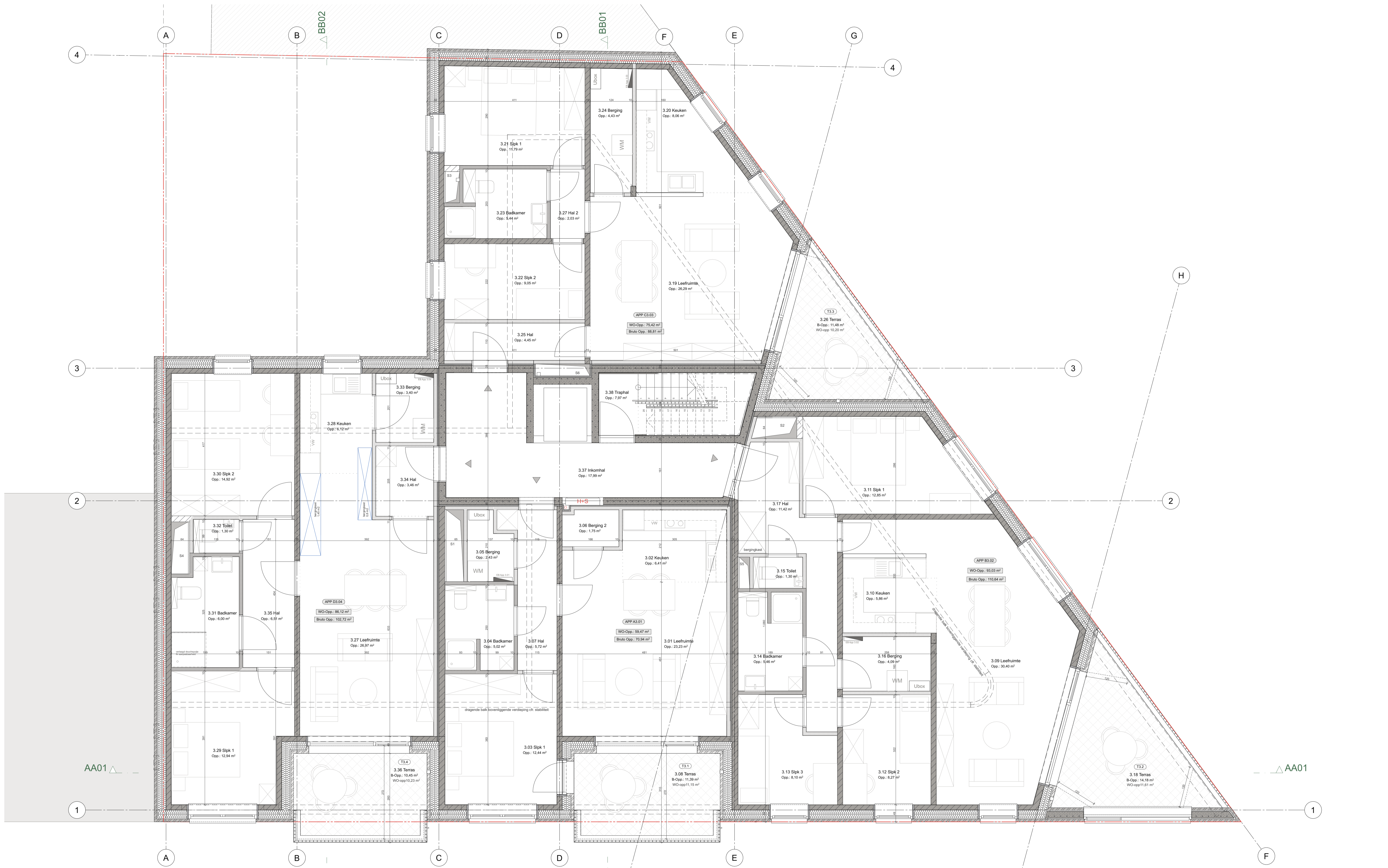
Plan +03 1:50 maatvoering cm
