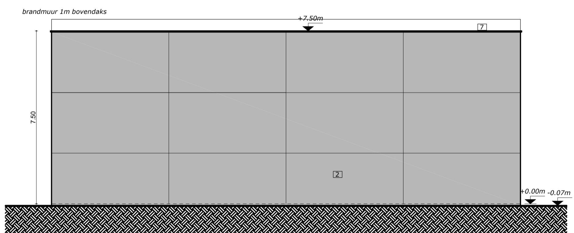
RECHTER GEVEL Bestaand BLOK 8
