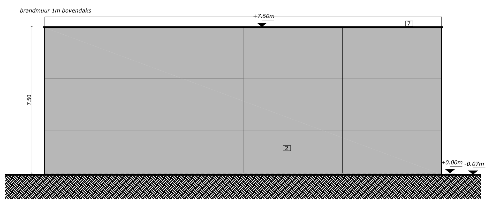
RECHTER GEVEL SCHAAL 1:100 BLOK 8 Vergunde toestand OMV referentie 2021132032 - 28.10.2021
