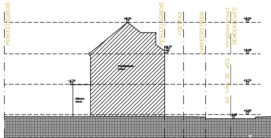
TERREINPROFIEL BT - schaal 1/200
