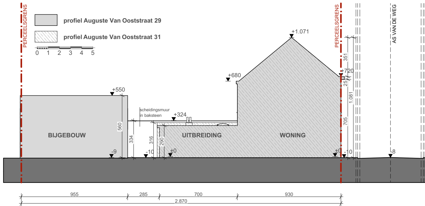
Terreinprofiel rechts - vergunde toestand schaal: 1/50
