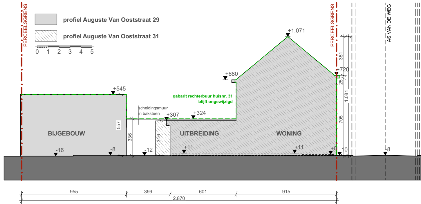
Terreinprofiel rechts - bestaande toestand schaal: 1/50
