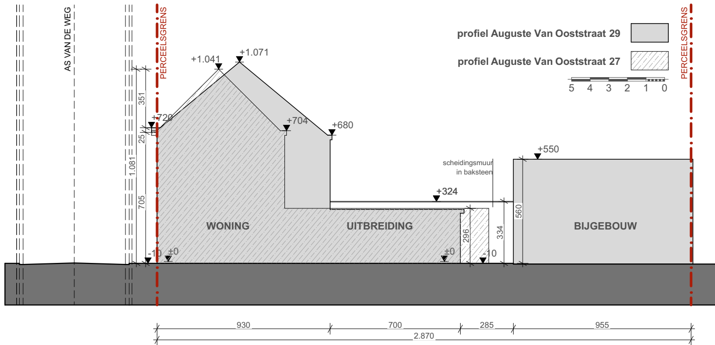
Terreinprofiel links - vergunde toestand schaal: 1/50
