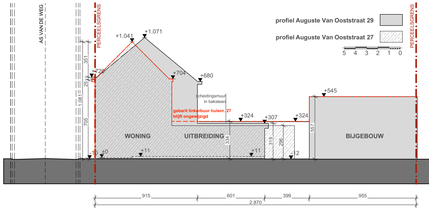
Terreinprofiel links - bestaande toestand schaal: 1/50
