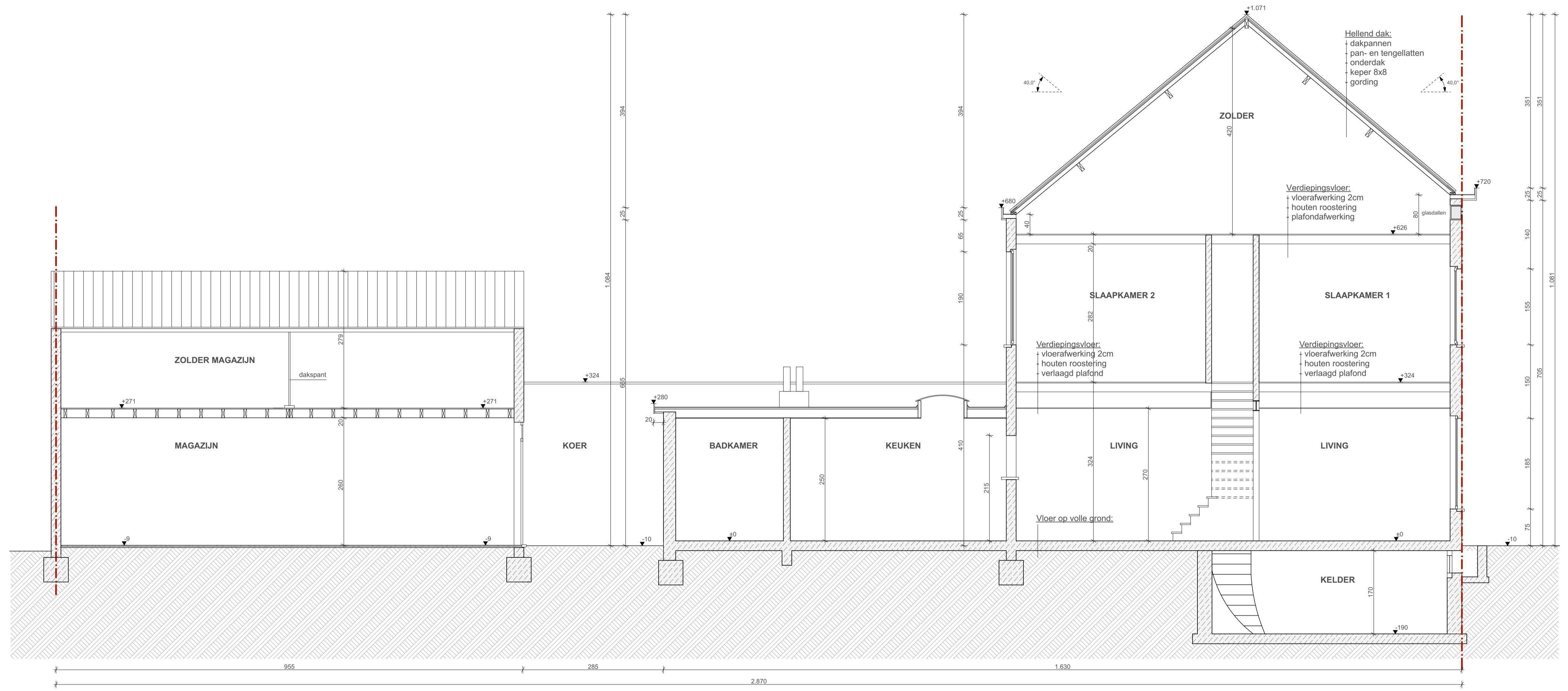
Doorsnede A - vergunde toestand schaal: 1/50
