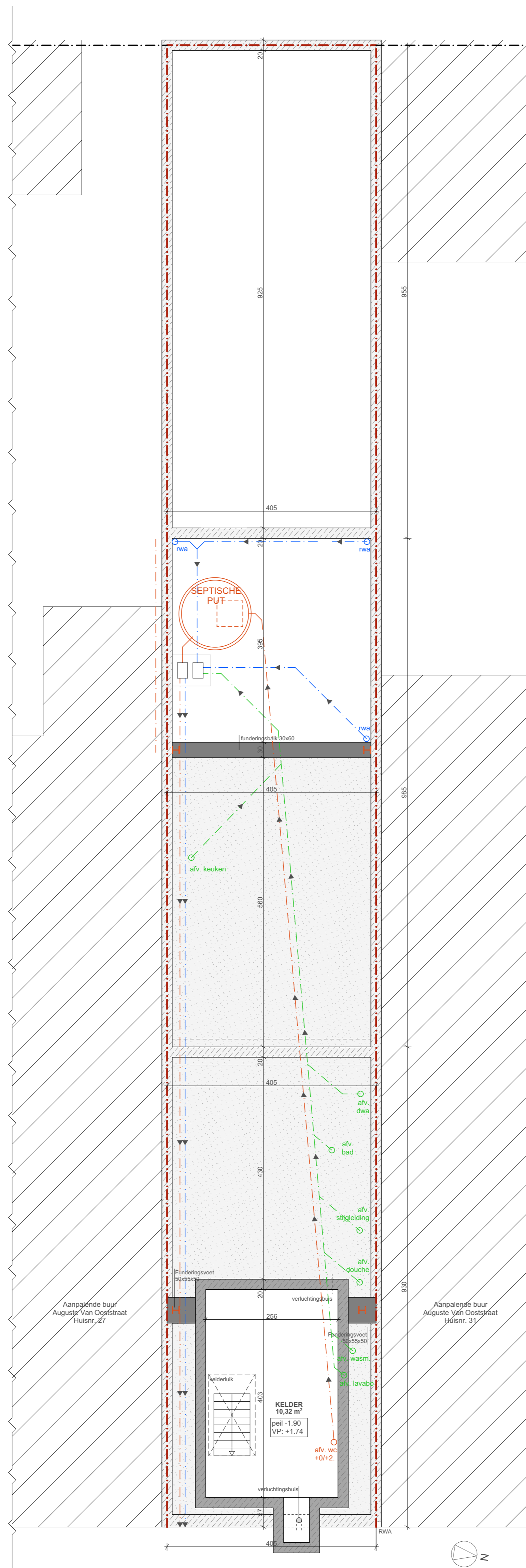
Fundering - bestaande toestand schaal: 1/50
