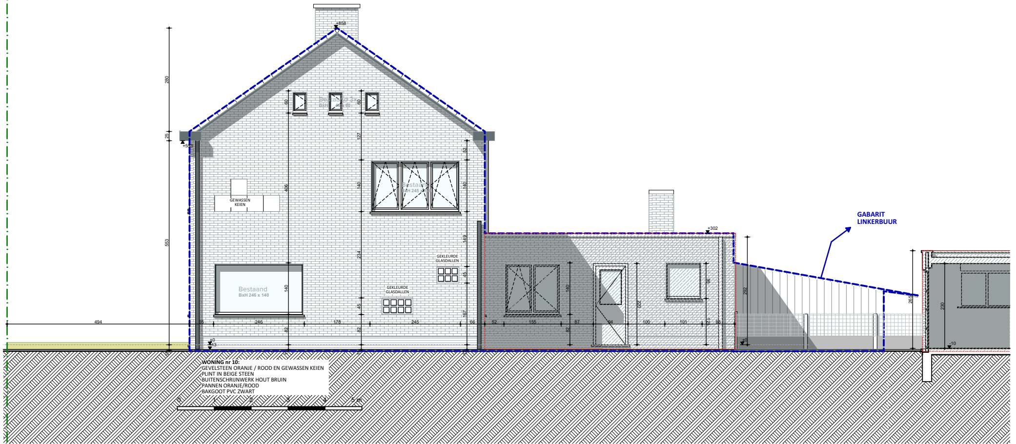
RECHTERGEVEL - Bestaande toestand
