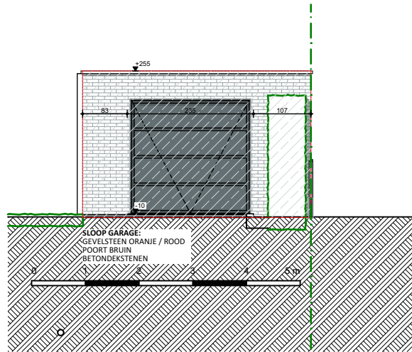
VOORGEVEL GARAGE SLOOP 1:100
